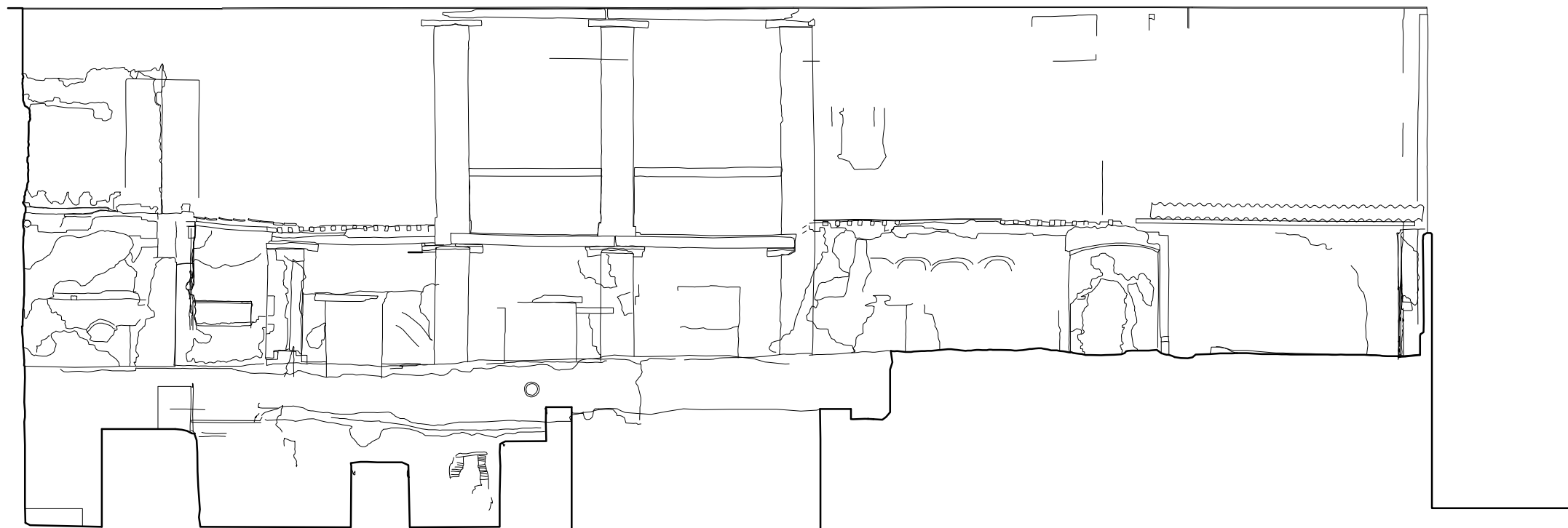
MARISTAN ESTADO ACTUAL SECCION TRANSVERSAL SUR A. ALMAGRO, A. ORIHUELA / arqs. ESCUELA DE ESTUDIOS ARABES, CSIC.
