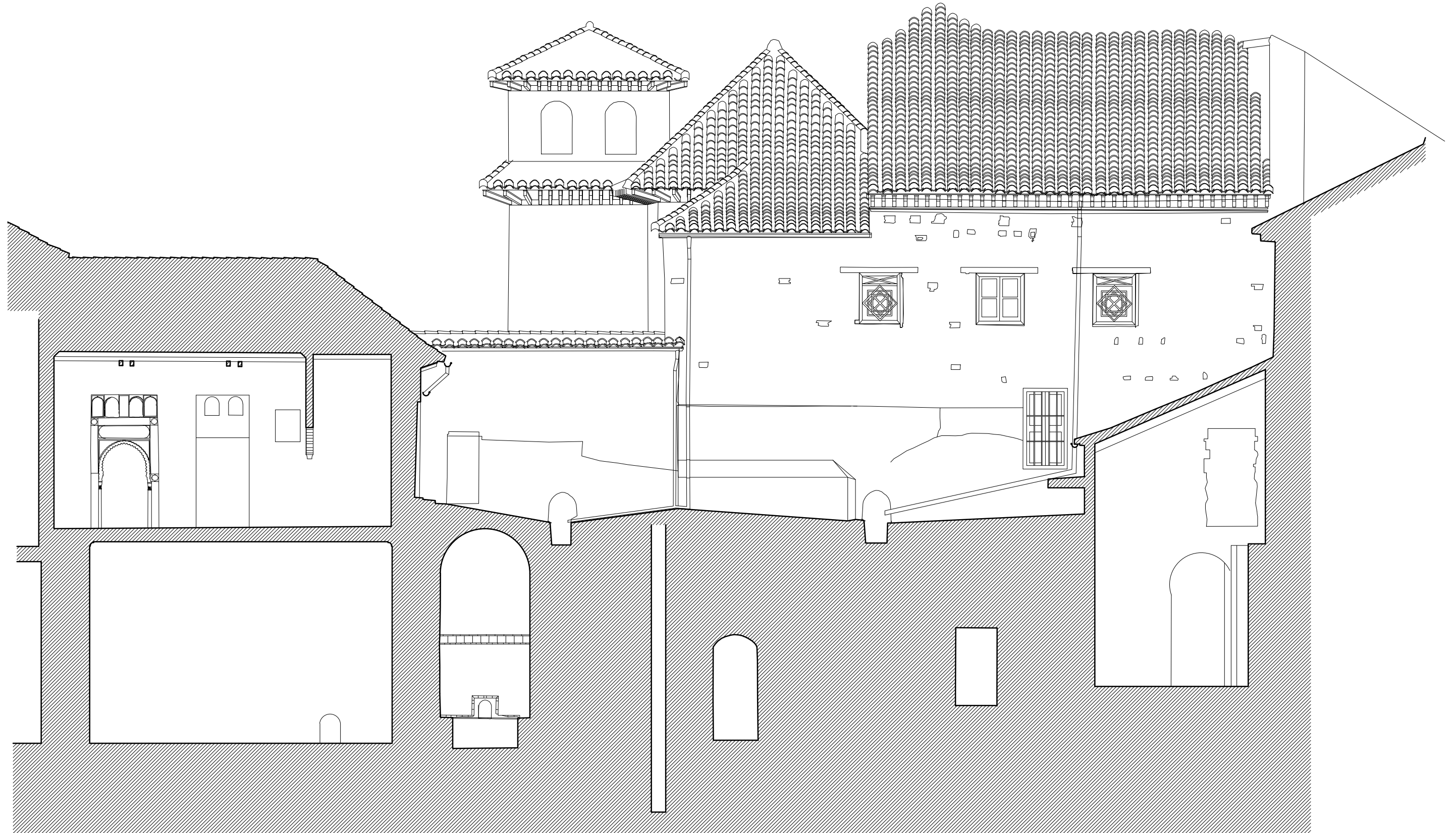
LA ALHAMBRA. HAMMAM DEL PALACIO DE COMARES. SECCIÓN N-S POR LETRINAS Y PILA FRÍA
