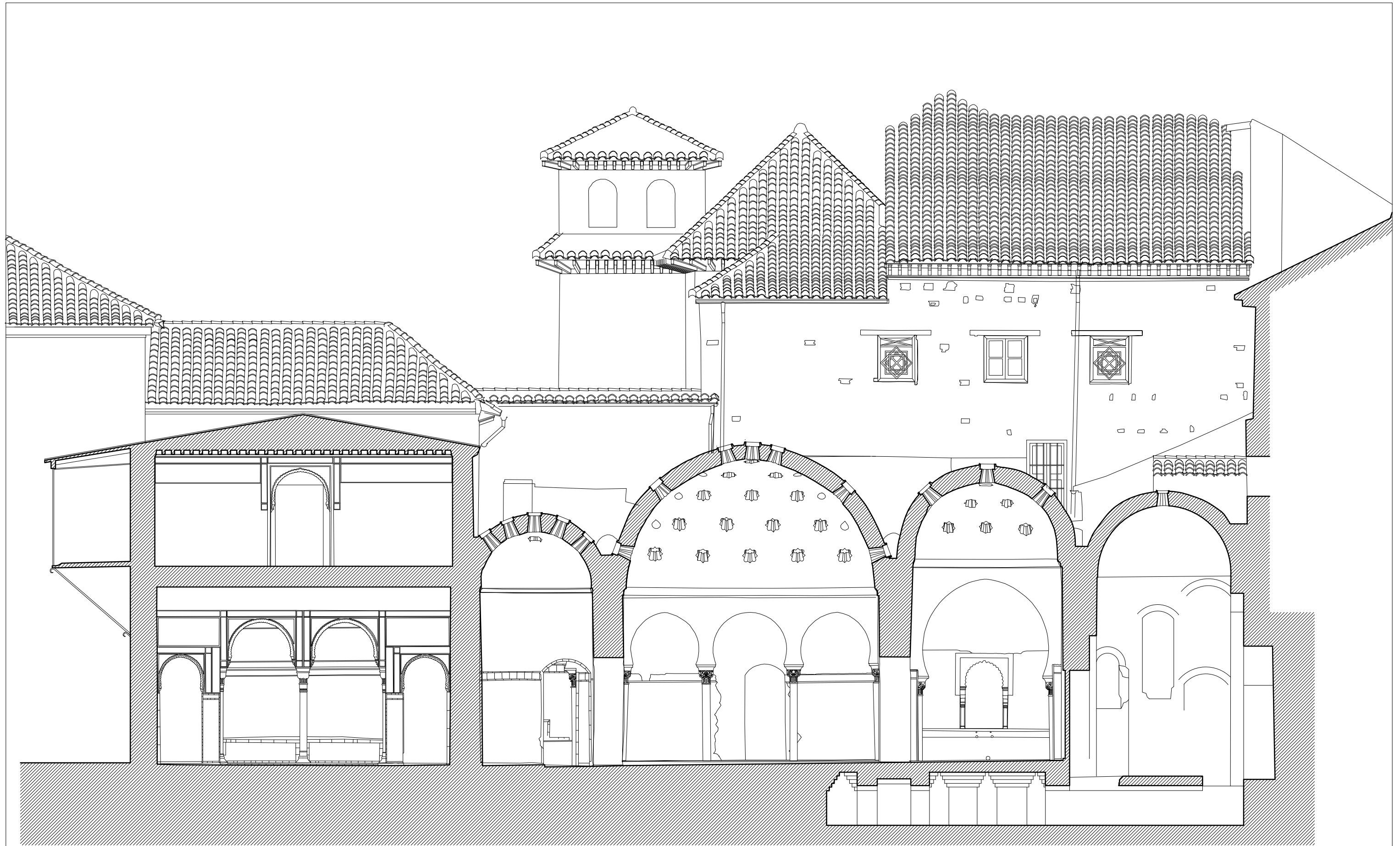
LA ALHAMBRA. HAMMAM DEL PALACIO DE COMARES. SECCIÓN N-S POR LATERAL DEL DAR AL-MAŠLAH
