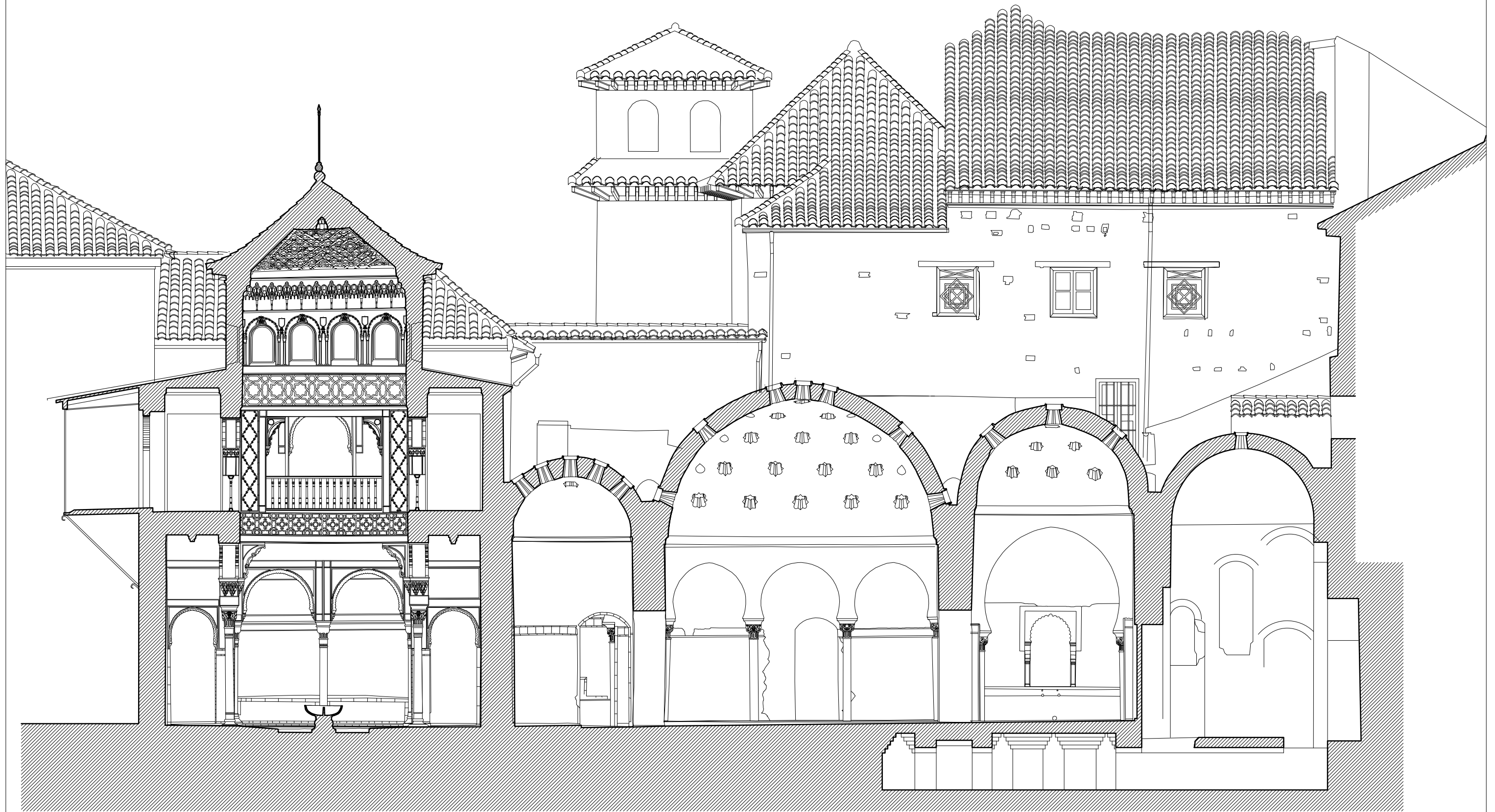
LA ALHAMBRA. HAMMAM DEL PALACIO DE COMARES. SECCIÓN N-S POR EL EJE DEL BAÑO
