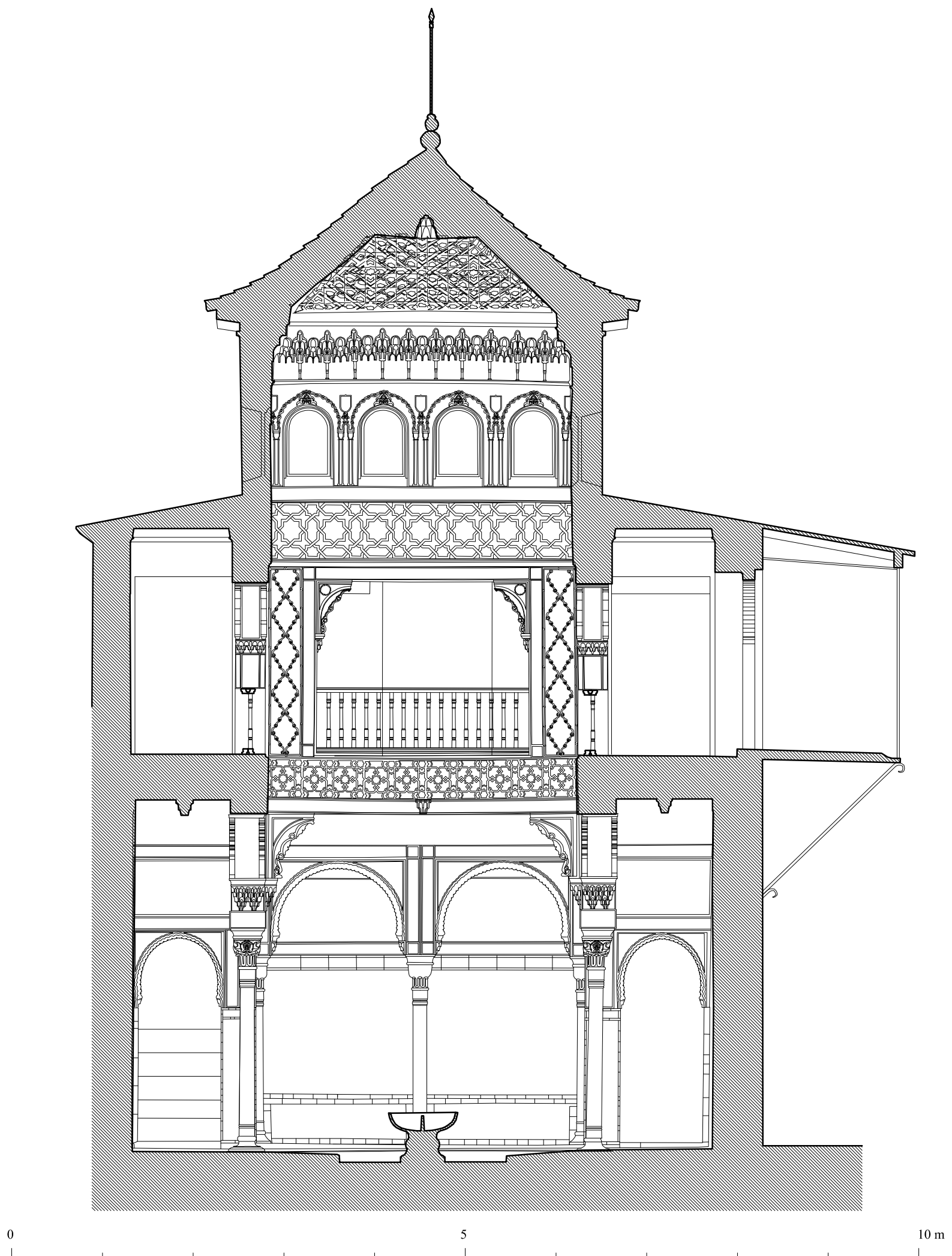
LA ALHAMBRA. HAMMAM DEL PALACIO DE COMARES. SECCIÓN S-N DEL DAR AL-MAŠLAH O SALA DE LAS CAMAS
