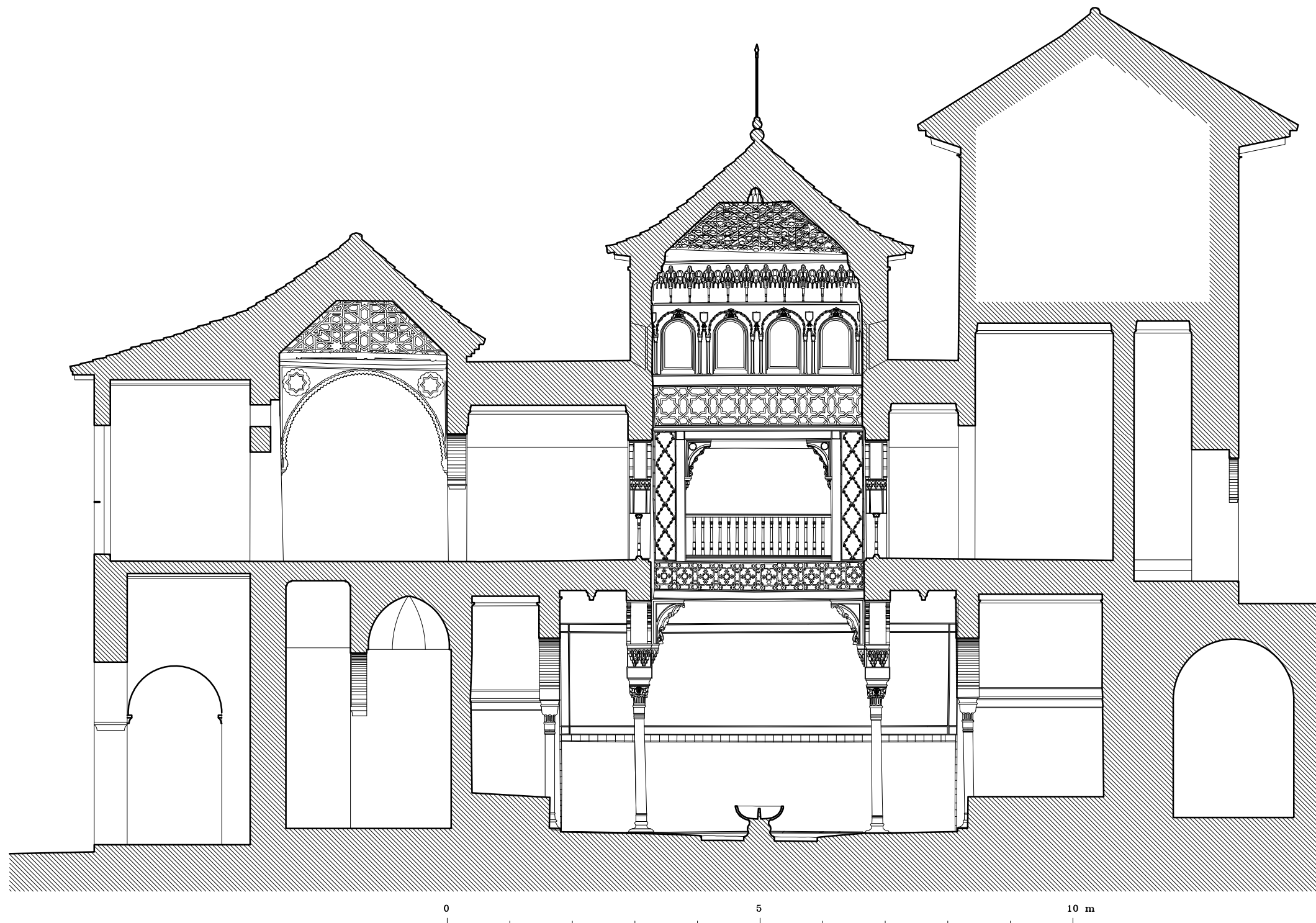
LA ALHAMBRA. HAMMAM DEL PALACIO DE COMARES. SECCIÓN E-O POR EL DAR AL-MAŠLAH O SALA DE LAS CAMAS
