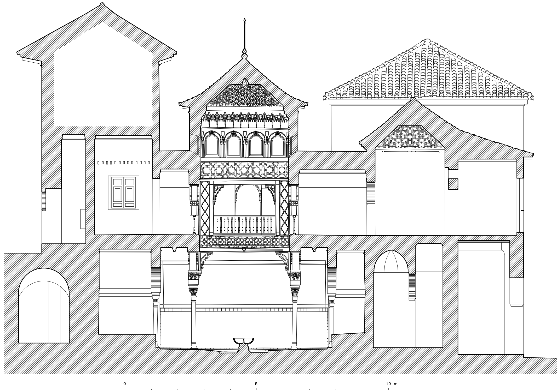
LA ALHAMBRA. HAMMAM DEL PALACIO DE COMARES. SECCIÓN O-E POR EL DAR AL-MAŠLAH
