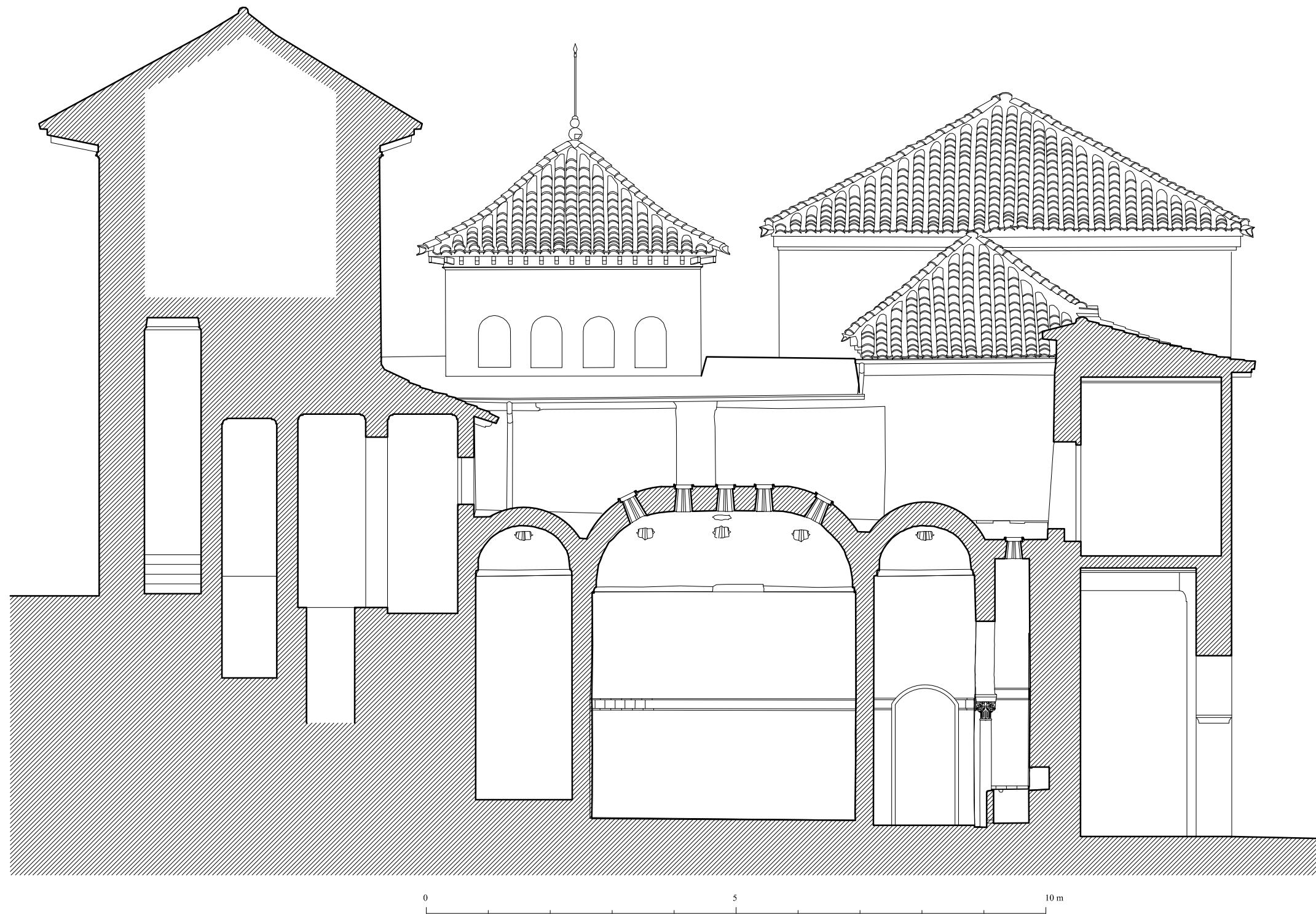
LA ALHAMBRA. HAMMAM DEL PALACIO DE COMARES. SECCIÓN O-E POR AL-BAYT AL-BARID
