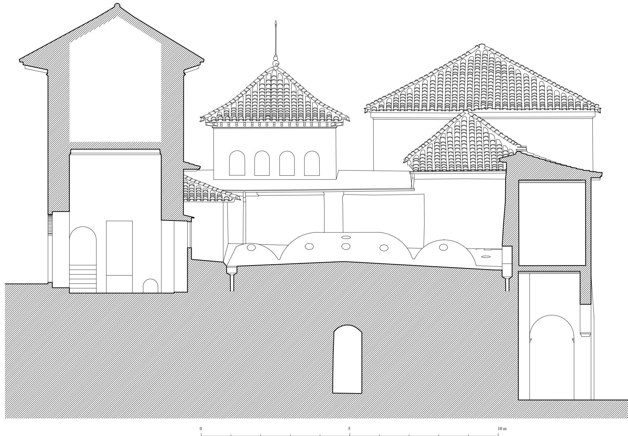
LA ALHAMBRA. HAMMAM DEL PALACIO DE COMARES. SECCIÓN O-E POR PASO ENTRE SALAS FRIA Y TEMPLADA
