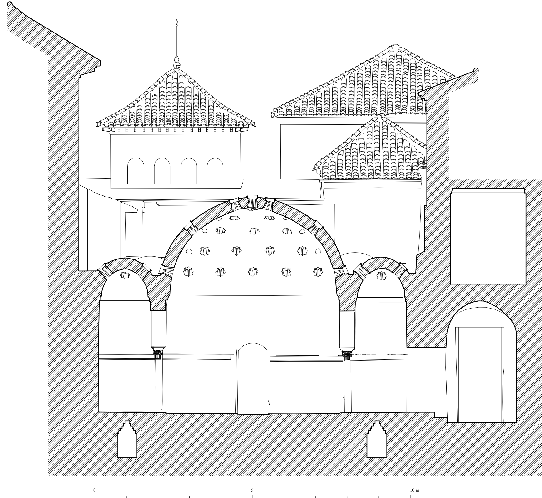
LA ALHAMBRA. HAMMAM DEL PALACIO DE COMARES. SECCIÓN O-E POR AL-BAYT AL-WASTANI
