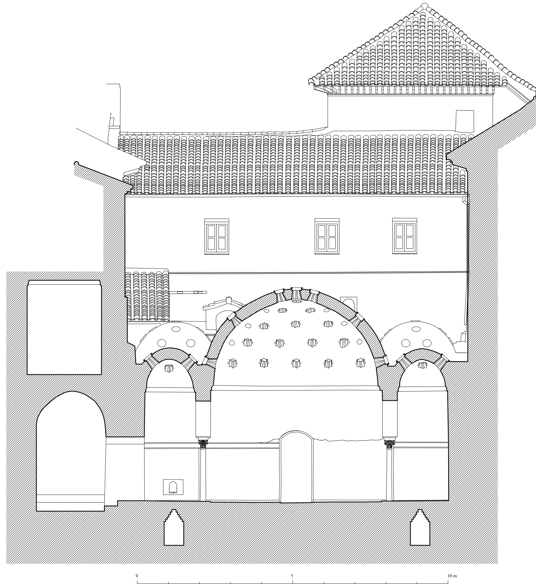
LA ALHAMBRA. HAMMAM DEL PALACIO DE COMARES. SECCIÓN E-O POR AL-BAYT AL-WASTANI
