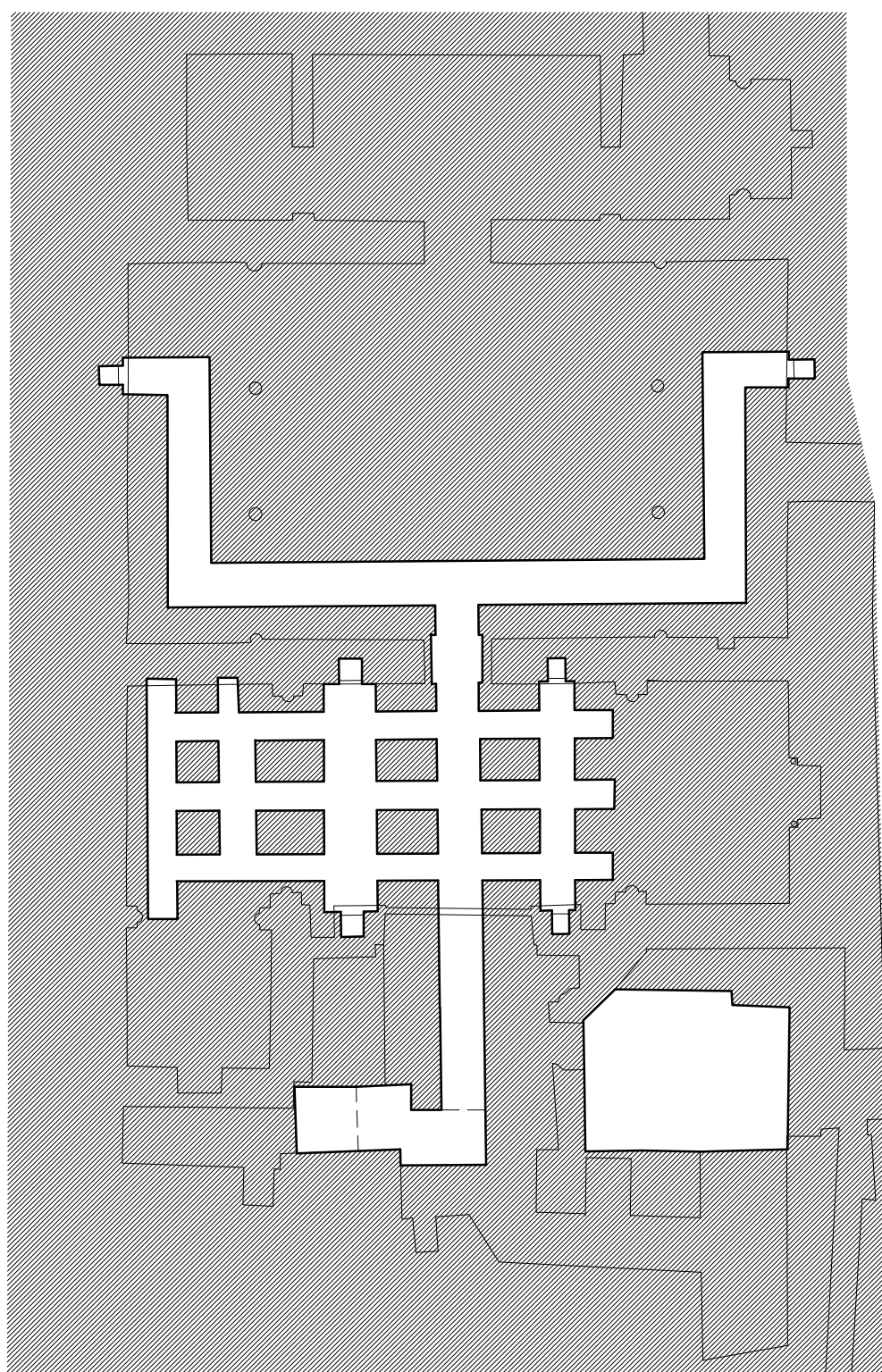
LA ALHAMBRA. HAMMAM DEL PALACIO DE COMARES. PLANTA DEL HIPOCAUSTO
