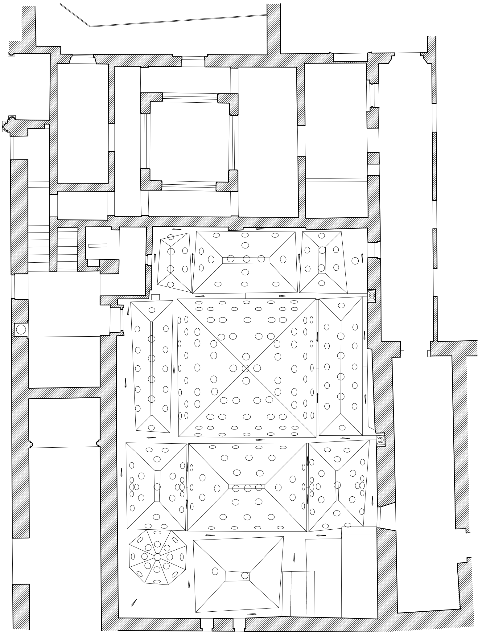
LA ALHAMBRA. HAMMAM DEL PALACIO DE COMARES. PLANTA ALTA
