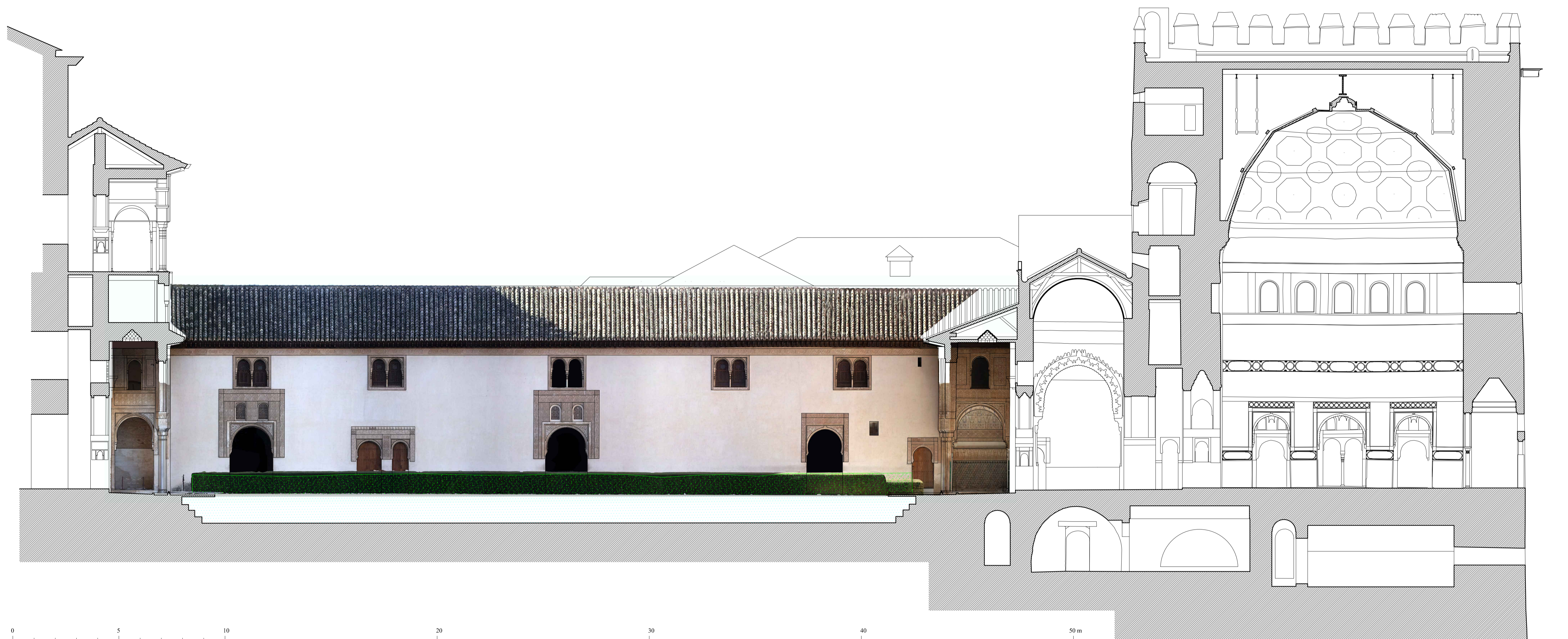
ALHAMBRA. PALACIO DE COMARES. SECCION HACIA OESTE.
