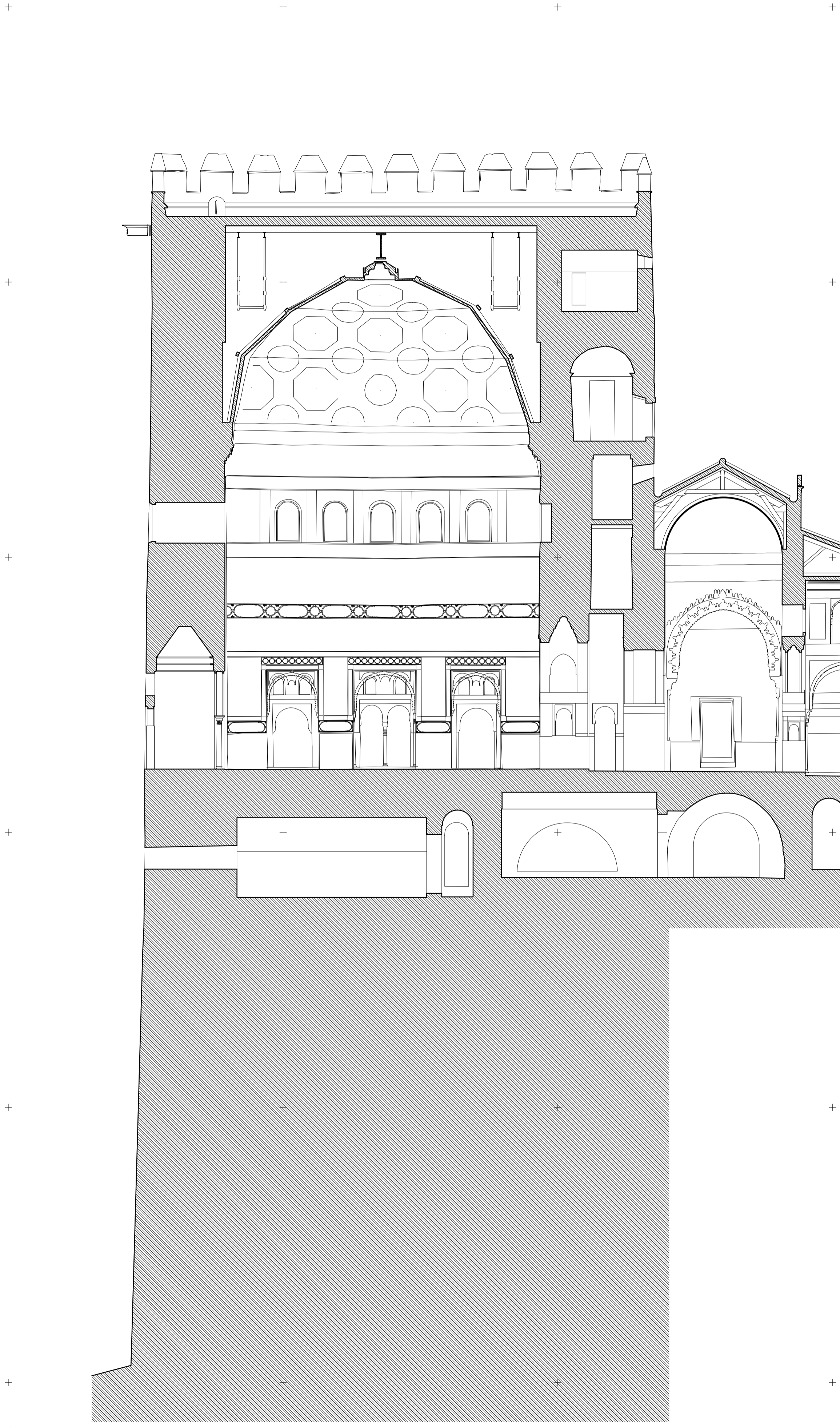
TORRE DE COMARES. LA ALHAMBRA. SECCION HACIA ESTE.
