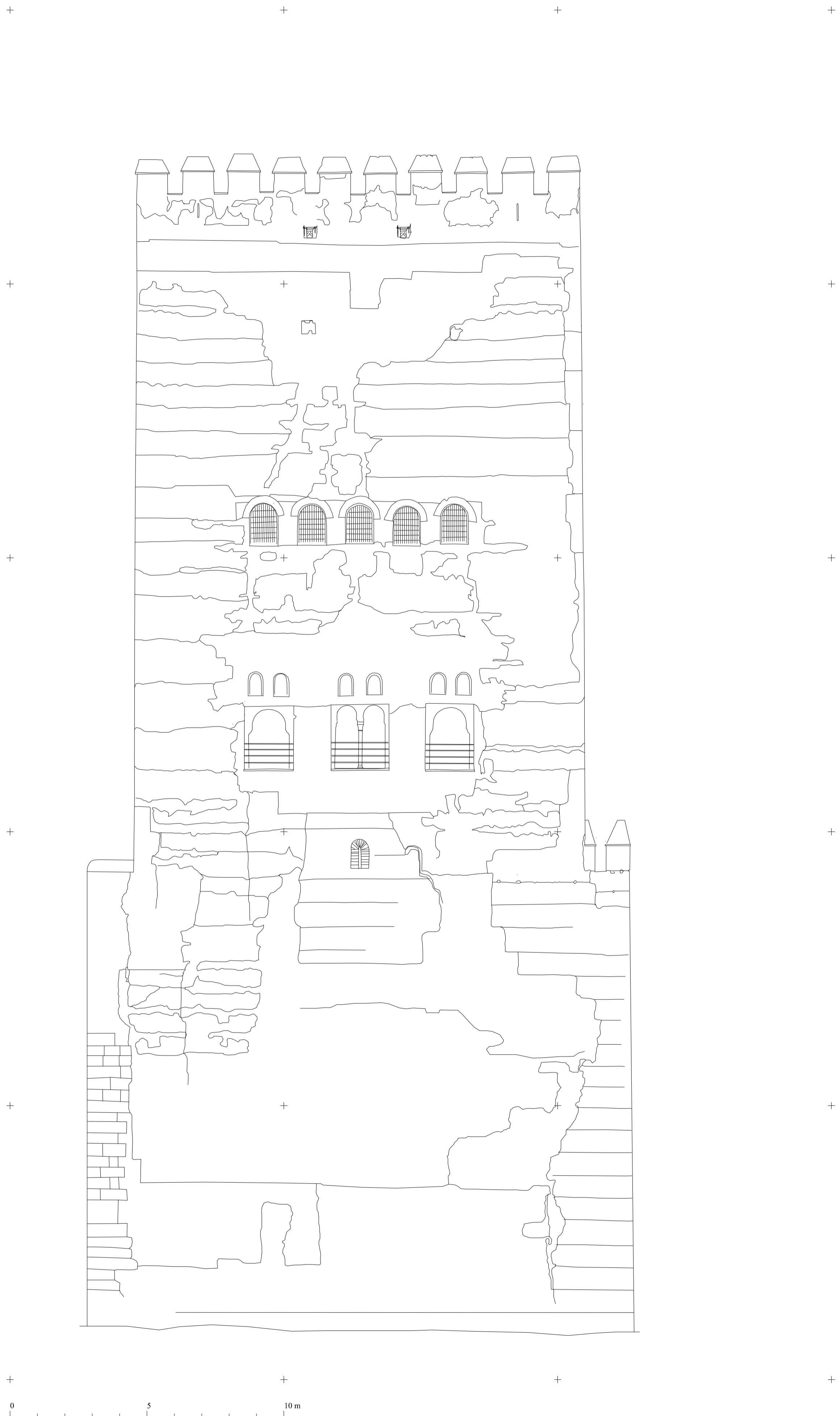
TORRE DE COMARES. LA ALHAMBRA. ALZADO NORTE.
