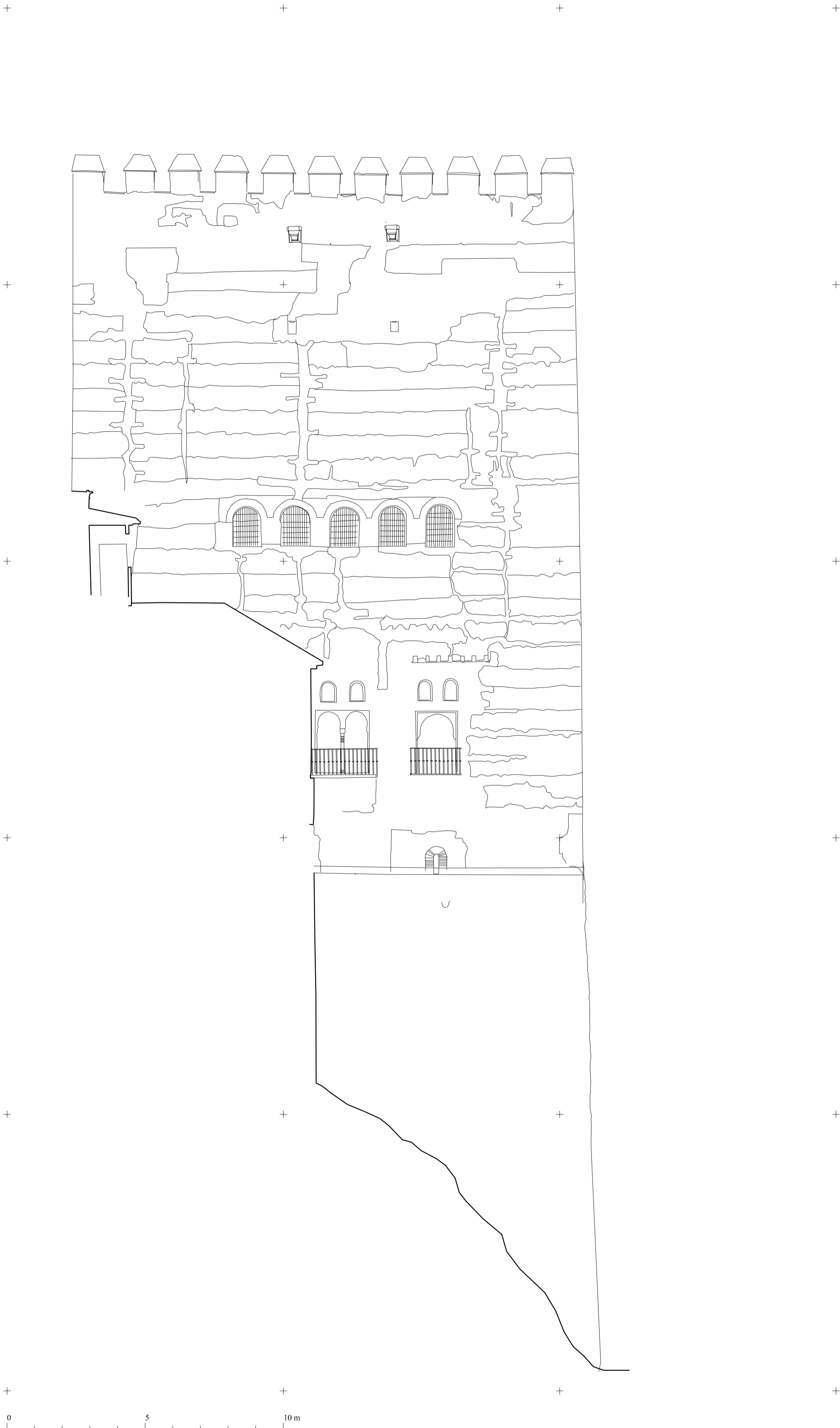
TORRE DE COMARES. LA ALHAMBRA. ALZADO ESTE.
