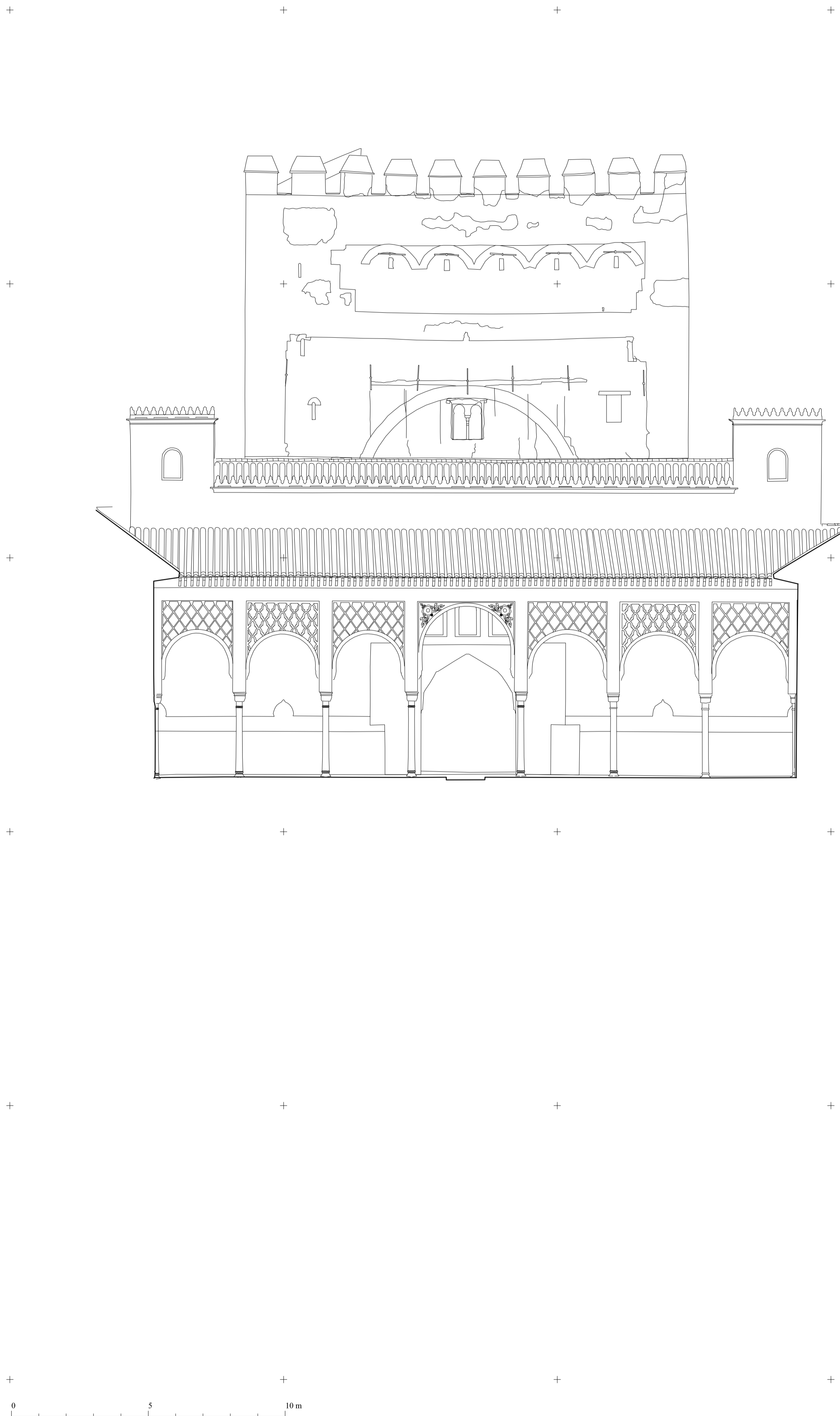
TORRE DE COMARES. LA ALHAMBRA. ALZADO SUR.
