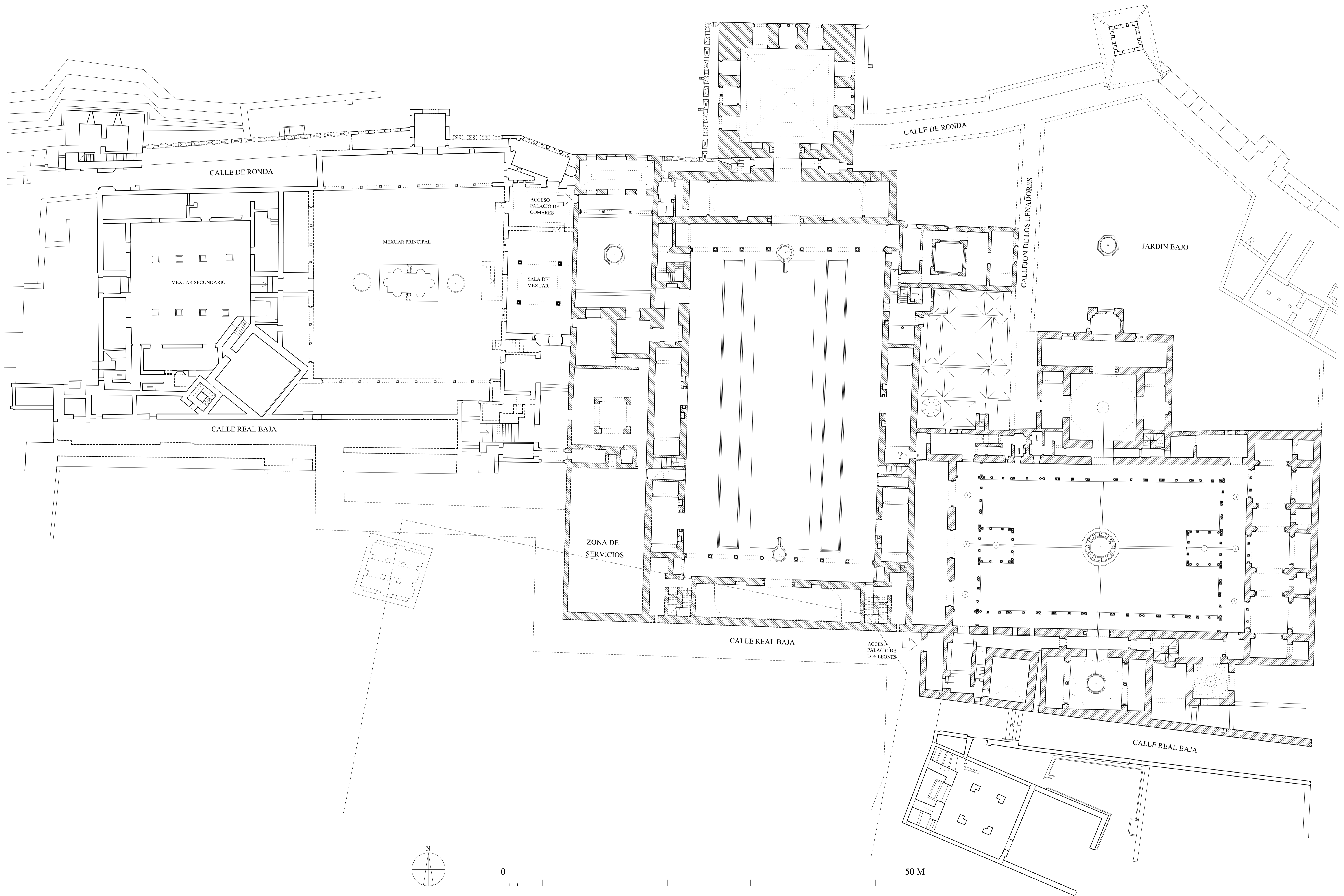
PALACIOS NAZARIES DE LA ALHAMBRA. GRANADA. (HIPOTESIS DE ESTADO INICIAL) ESCUELA DE ESTUDIOS ARABES. C.S.I.C. julio 1994. A.ORIHUELA/arq.
