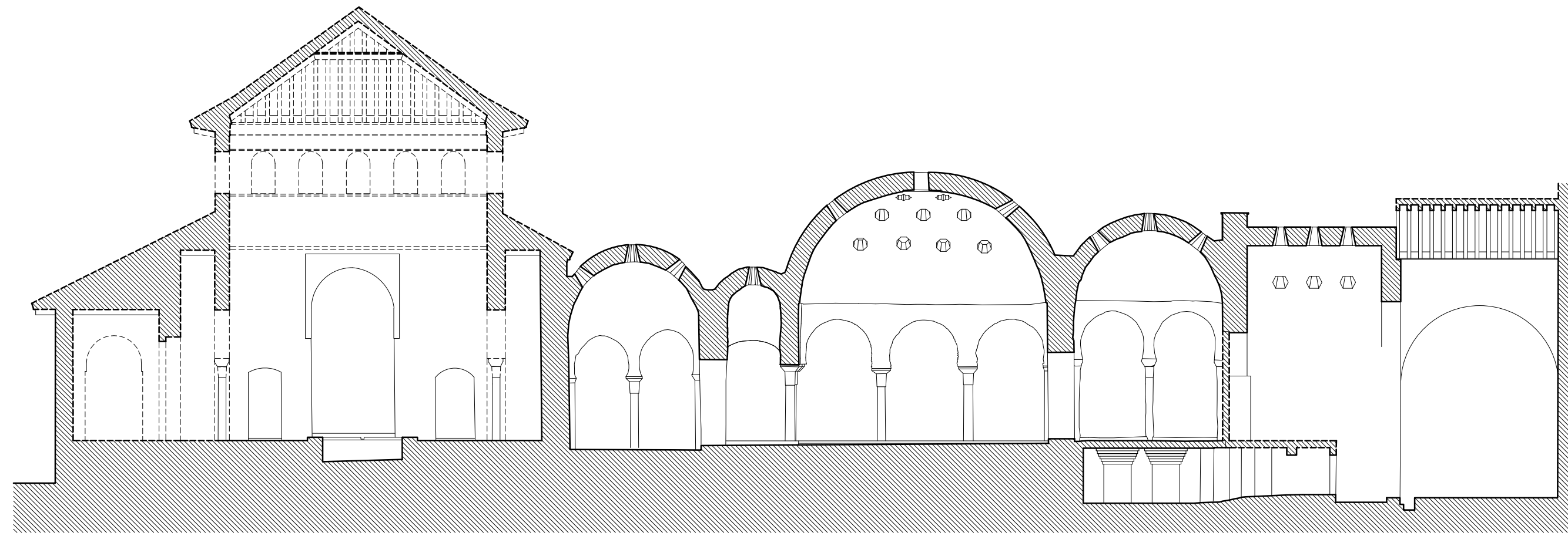
SECCION AA
