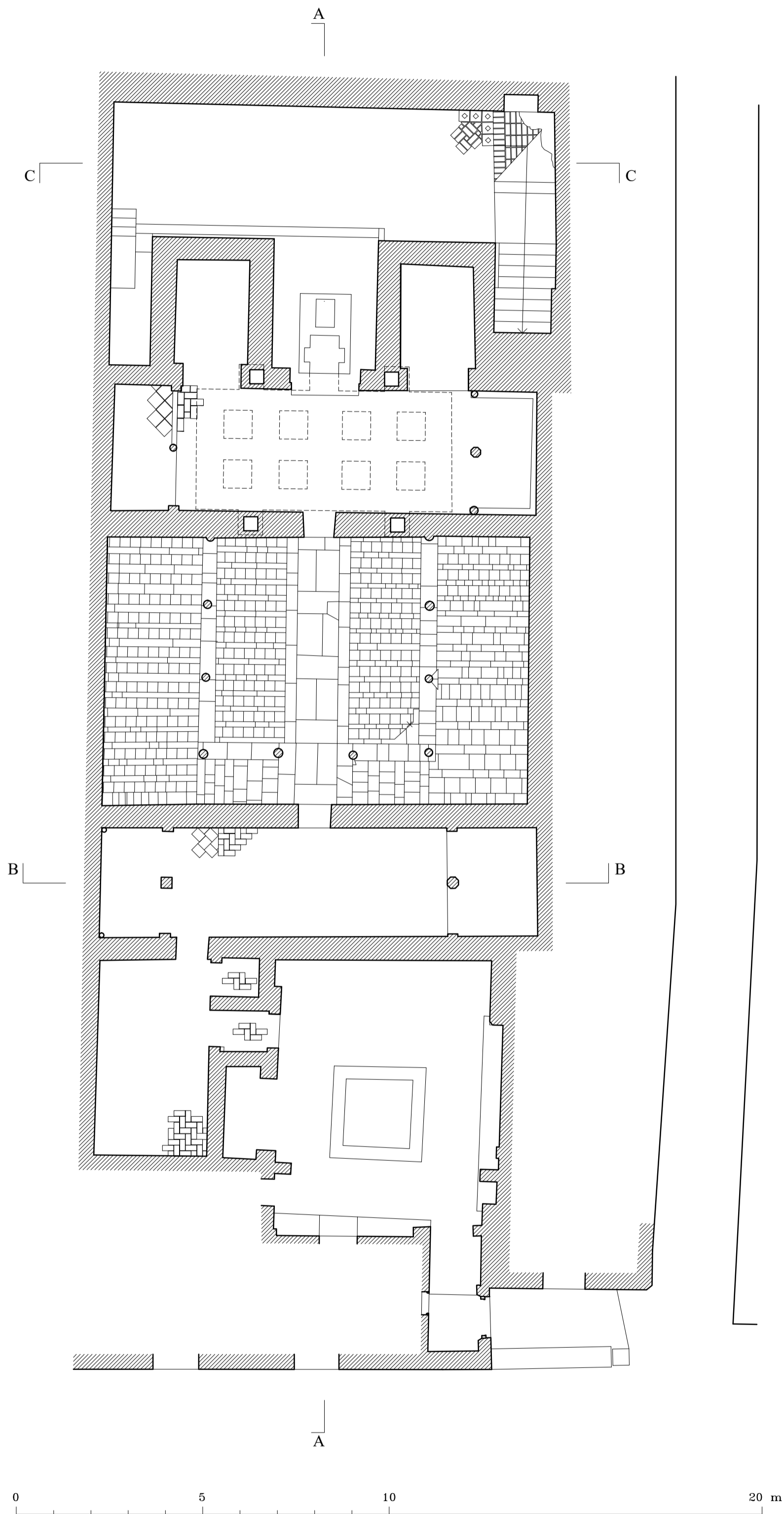
EL BAÑUELO (HAMMAM AL-YAWZ). GRANADA. PLANTA ESCUELA DE ESTUDIOS ARABES. C.S.I.C. A. ALMAGRO/arq.
