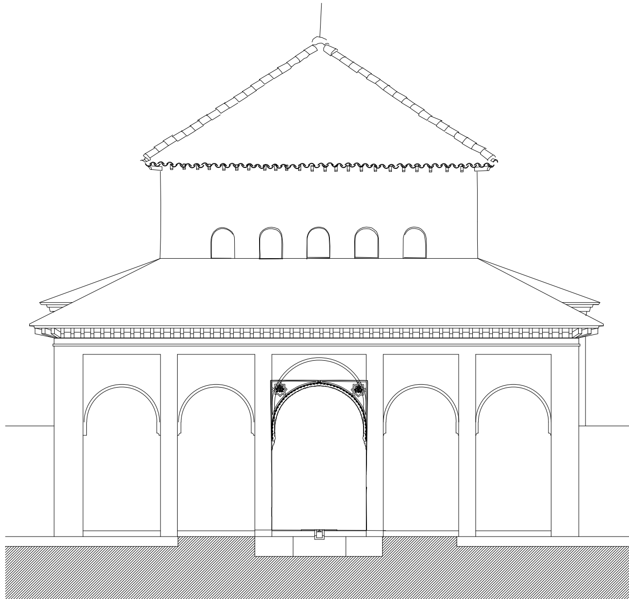
CUARTO REAL DE SANTO DOMINGO PROPUESTA ALZADO NORTE ESCUELA DE ESTUDIOS ARABES. C.S.I.C. A.ALMAGRO/arq, A. ORIHUELA/arq.
