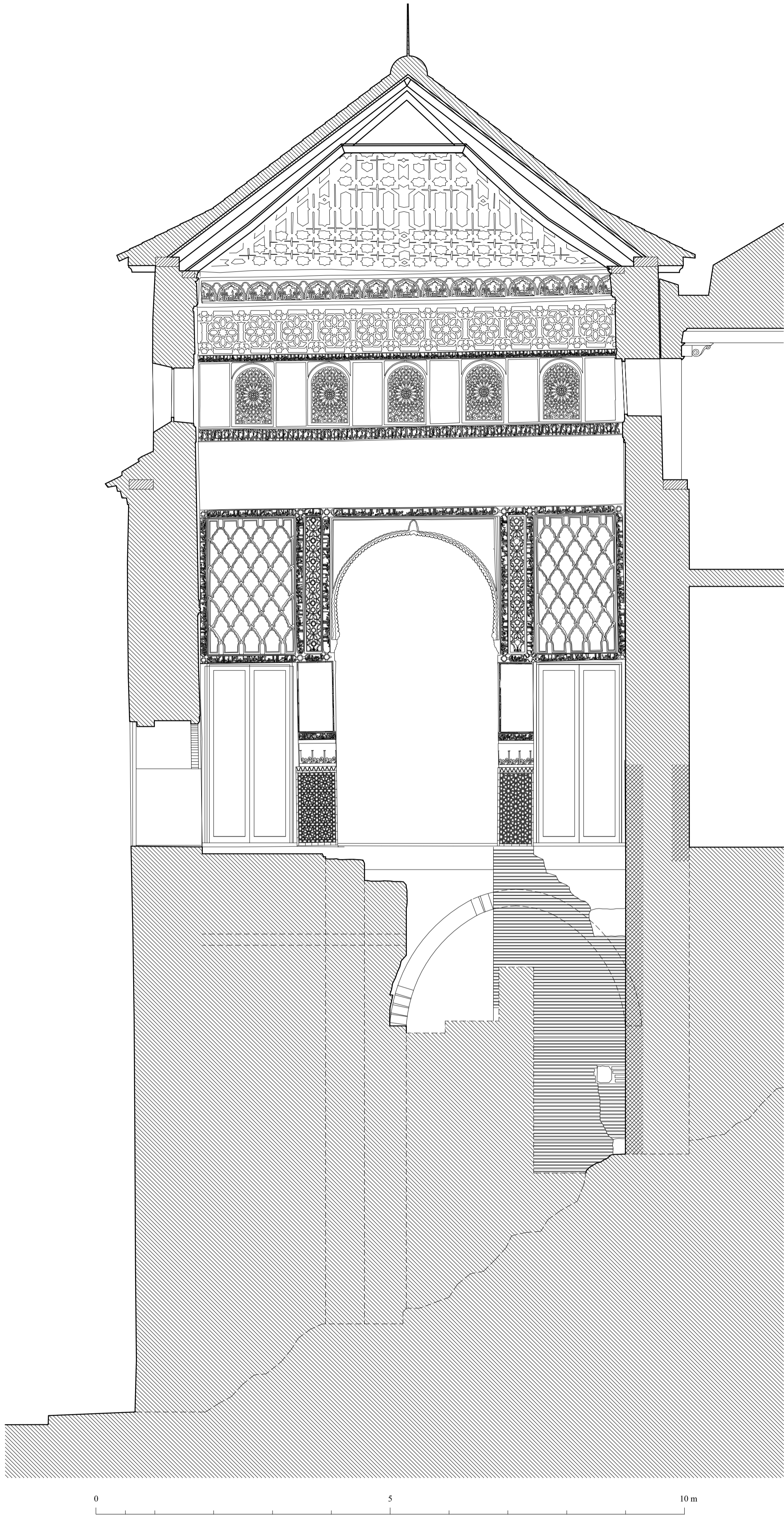
CUARTO REAL DE SANTO DOMINGO. GRANADA. SECCION DE LA EXCAVACIÓN HACIA OESTE
