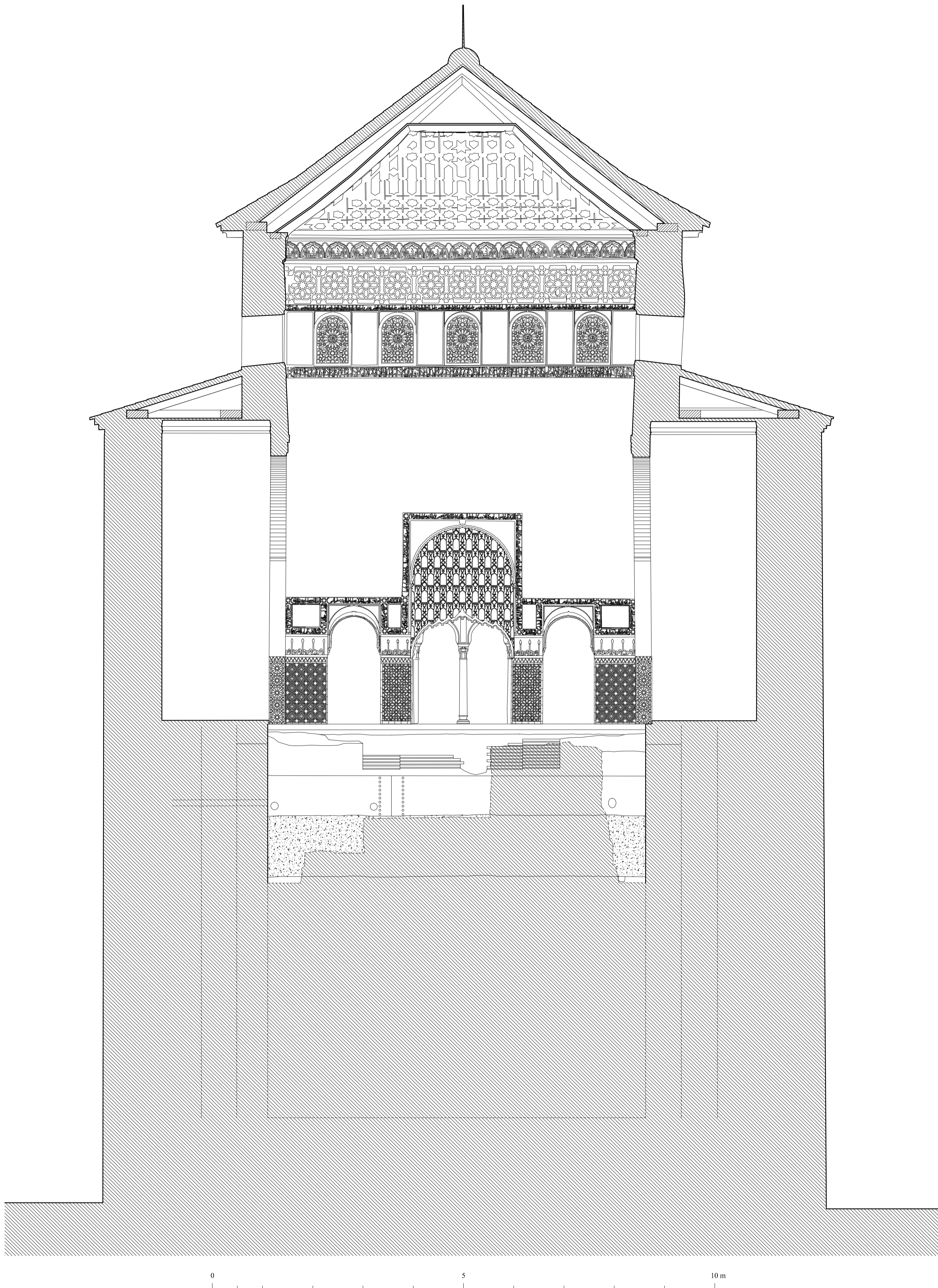
CUARTO REAL DE SANTO DOMINGO. GRANADA. SECCION DE LA EXCAVACIÓN HACIA SUR
