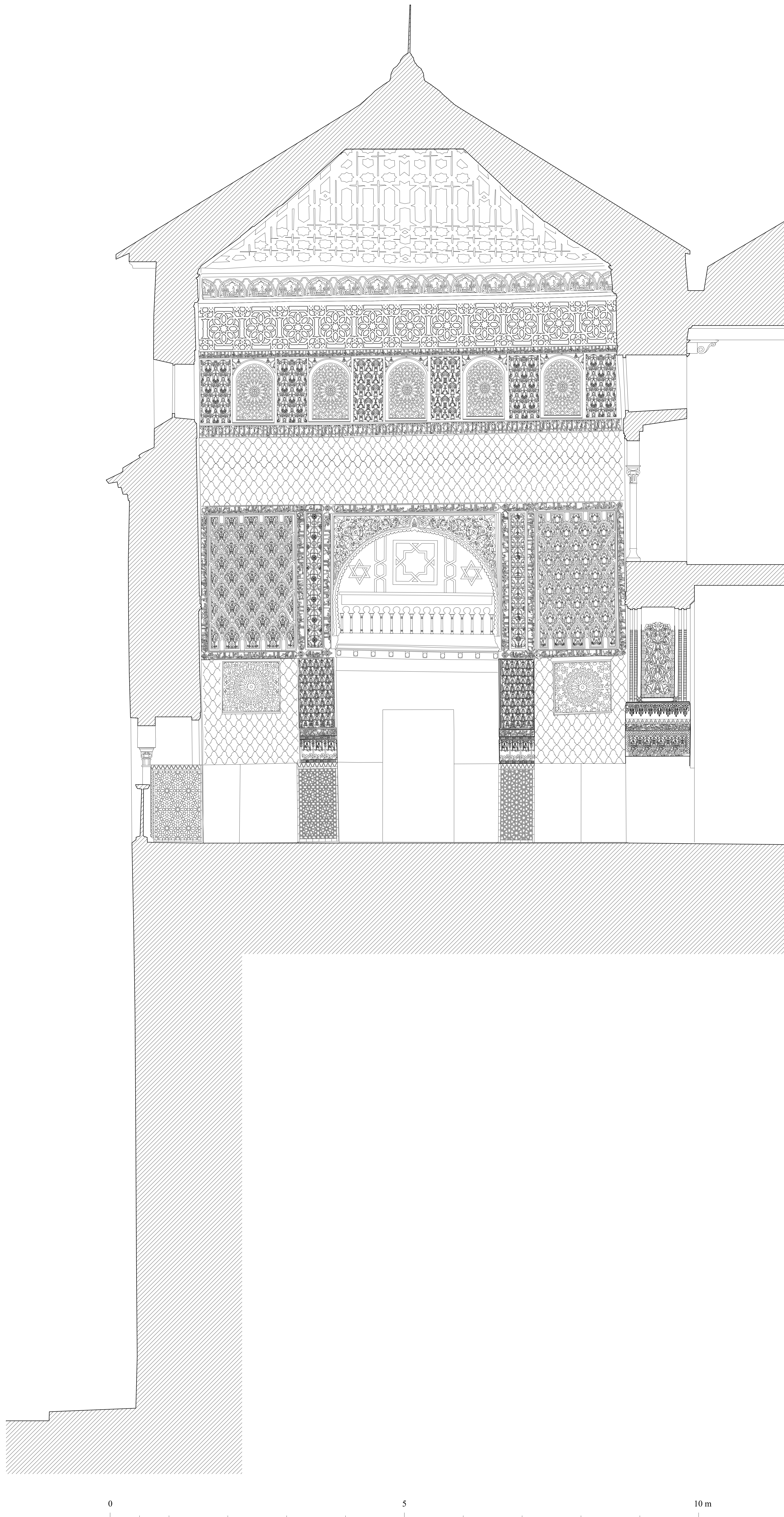
CUARTO REAL DE SANTO DOMINGO. GRANADA. SECCION DE LA QUBBA HACIA OESTE
