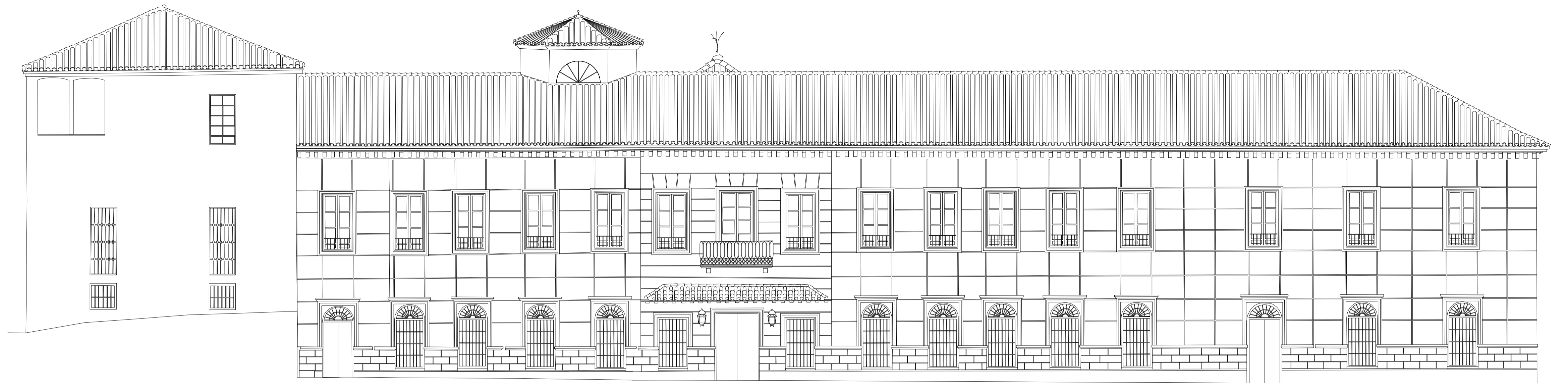
ALZADO NORTE
