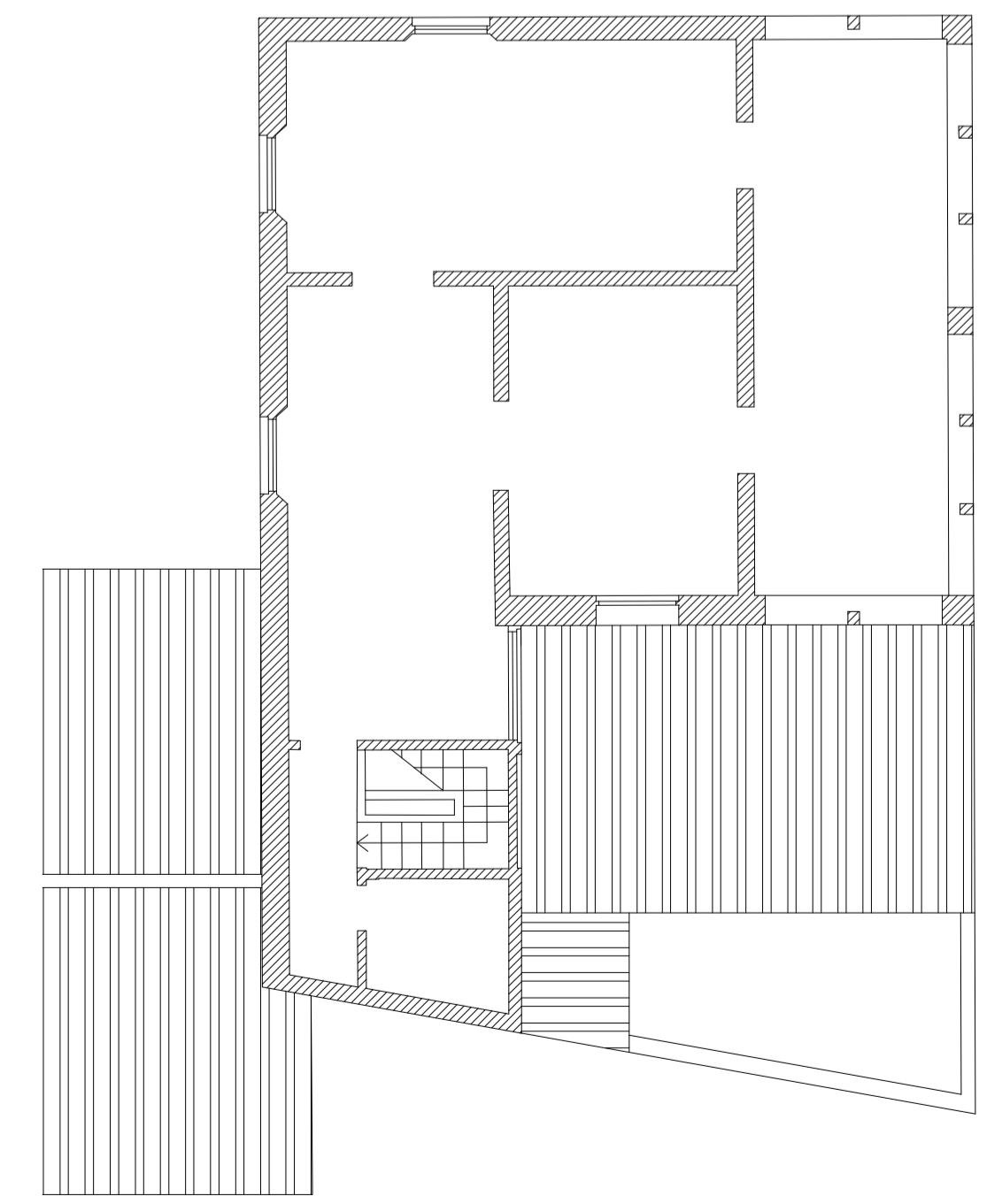
PLANTA TORREÓN
