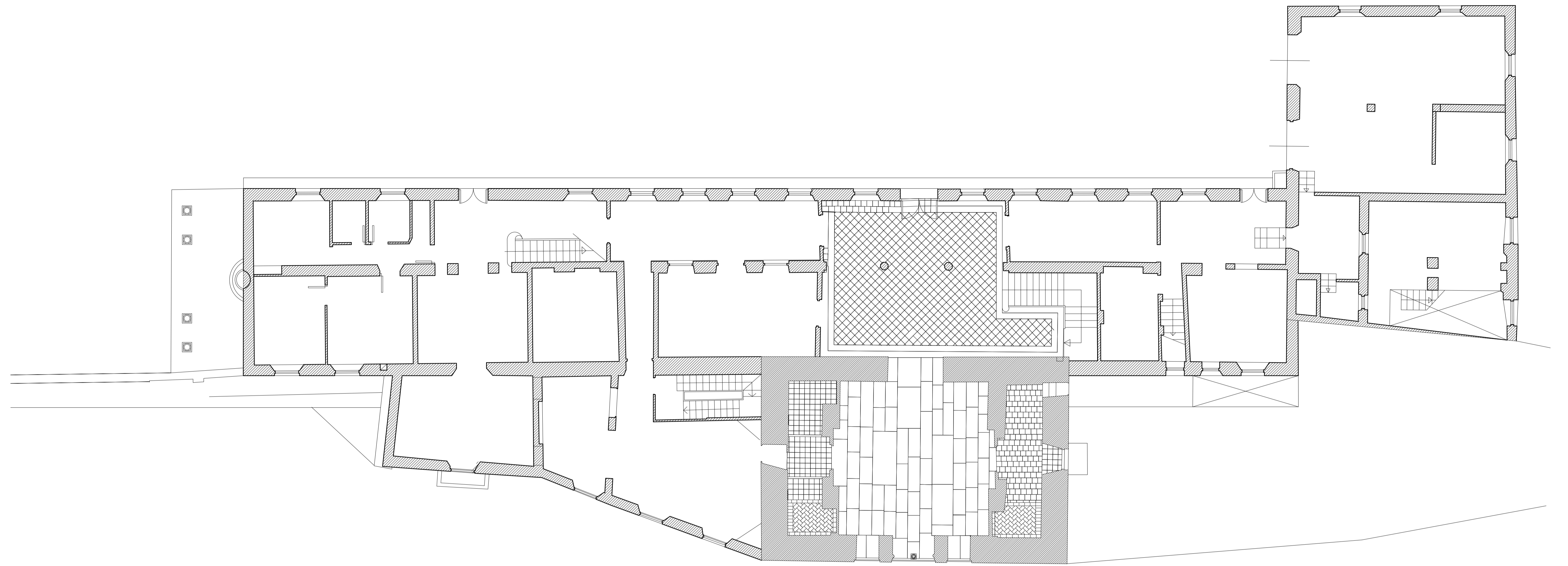
PLANTA BAJA
