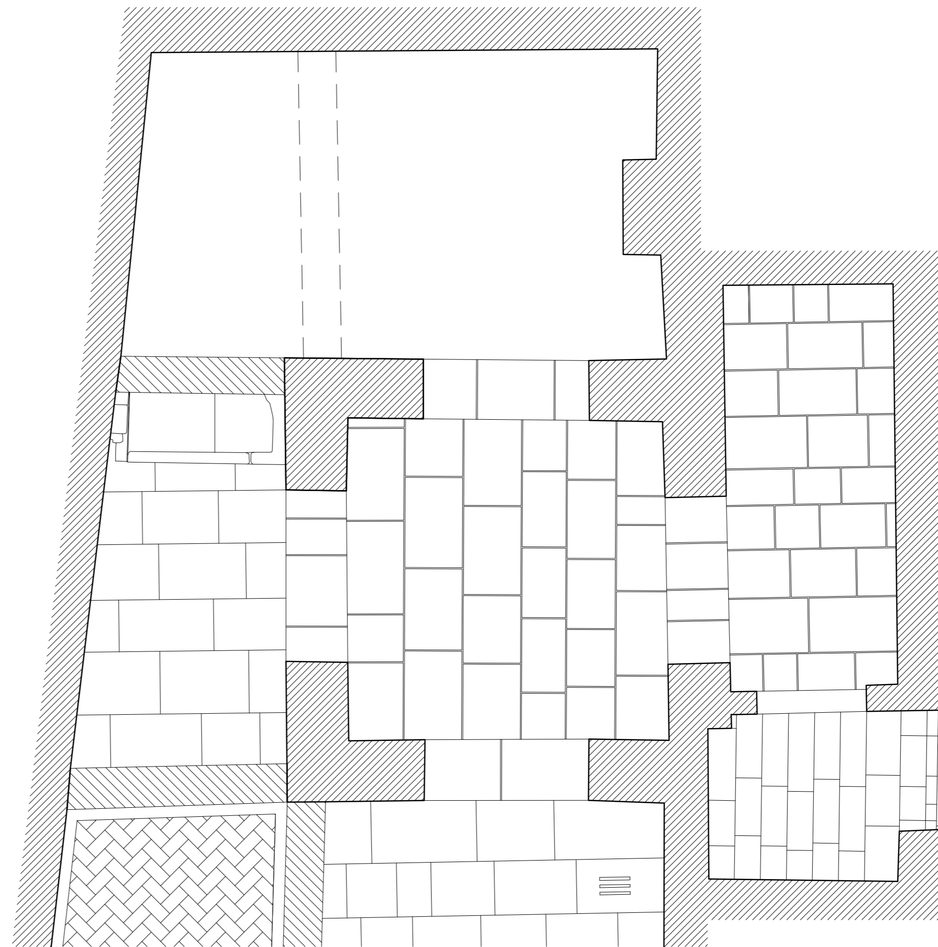
LA ALHAMBRA. GRANADA. QUBBA JUNTO A LA RAWDA PLANTAS BAJA, BOVEDA Y CUBIERTA
