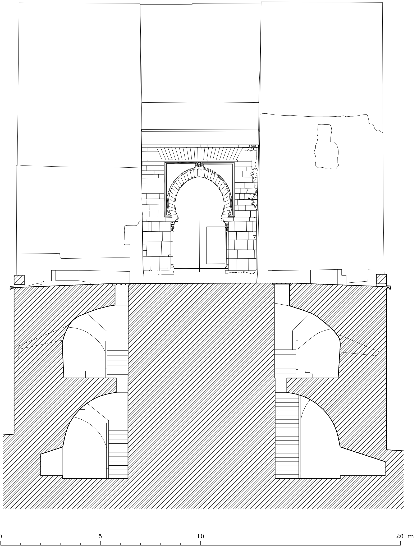
LA ALHAMBRA. PUERTA DE LOS SIETE SUELOS. ALZADO A. ALMAGRO /arq. ESCUELA DE ESTUDIOS ARABES, C.S.I.C.
