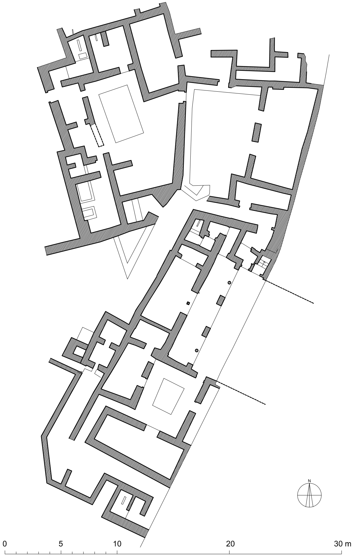
ALCAZABA DE SILVES ( PORTUGAL) PALACIO ALMOHADE Basado en planimetría de Rosa y Mario Varela Gomes
