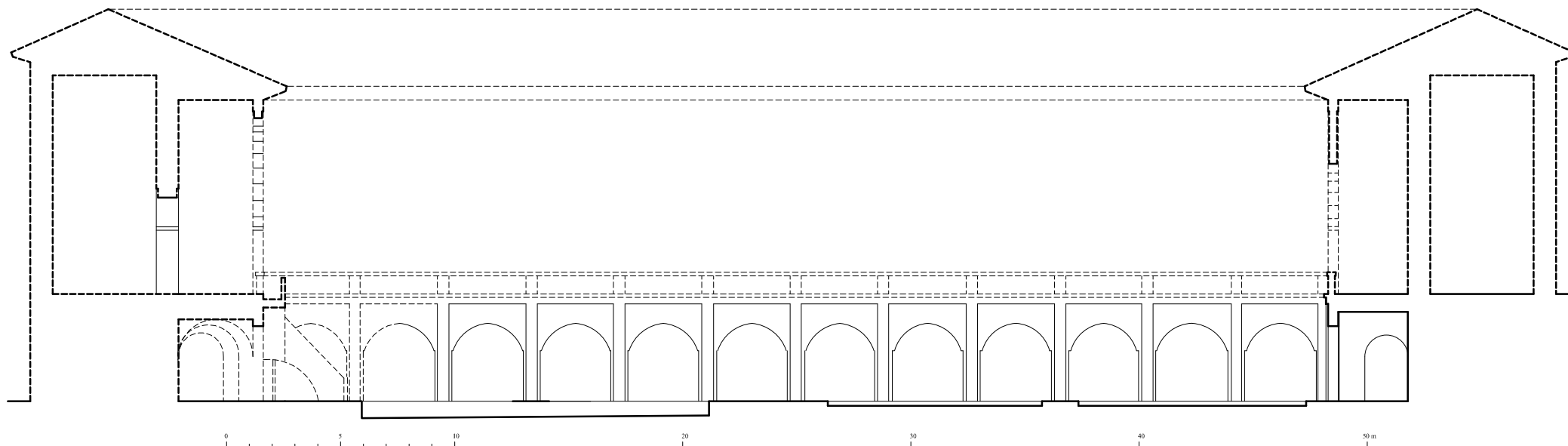
ALCAZAR DE SEVILLA. PATIO DEL CRUCERO. HIPÓTESIS DEL PATIO ISLÁMICO. ESCUELA DE ESTUDIOS ÁRABES, C.S.I.C. A. ALMAGRO o arq.
