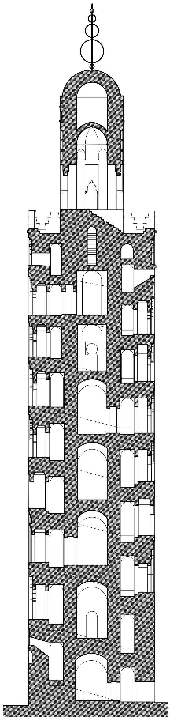
ALMINAR ALMOHADE DE SEVILLA. SECCION ESTE-OESTE. ESCUELA DE ESTUDIOS ARABES. A. ALMAGRO/arq.
