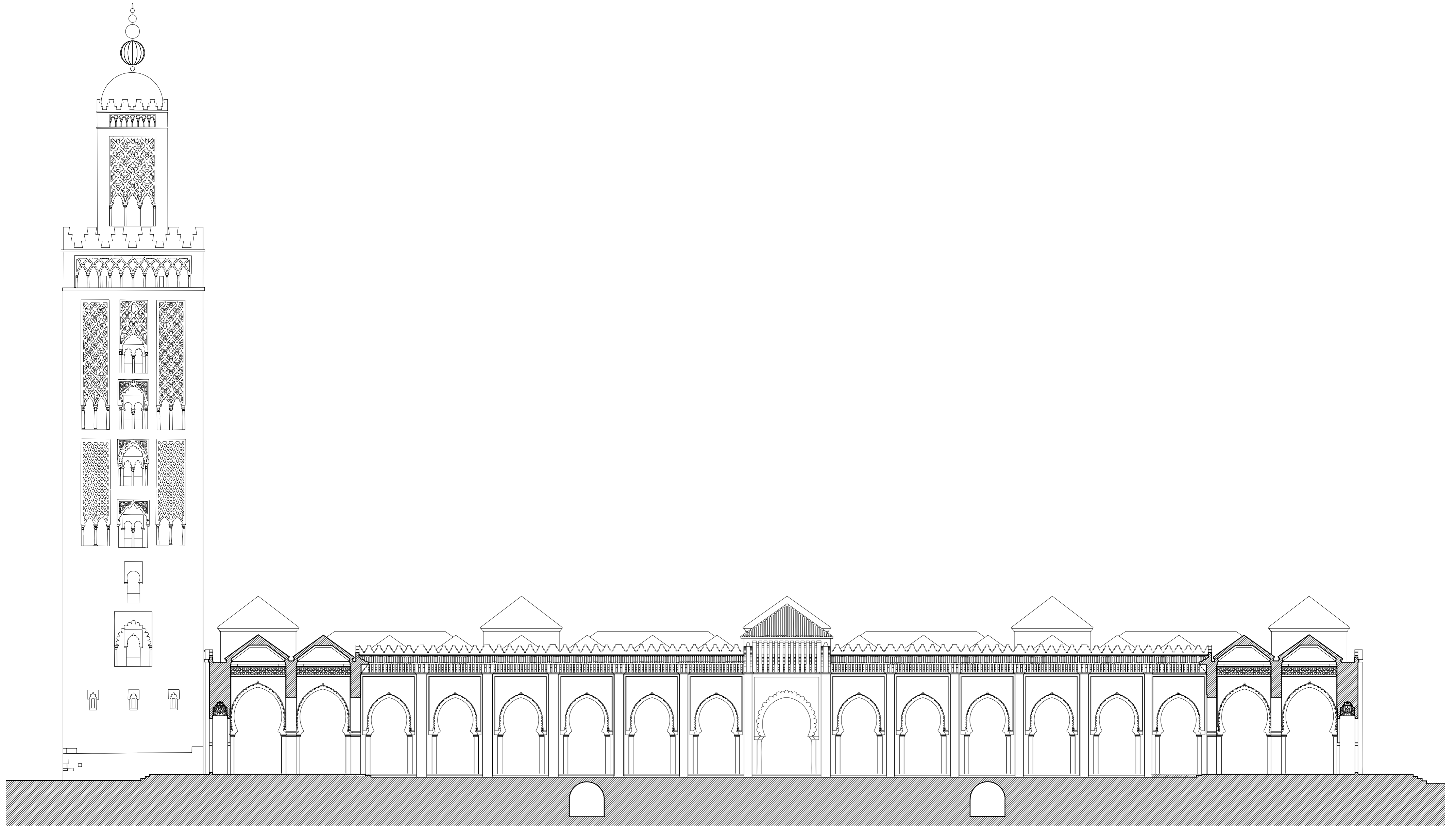
MEZQUITA ALMOHADE DE SEVILLA. SECCION TRANSVERSAL. ESCUELA DE ESTUDIOS ARABES. A. ALMAGRO arg.
