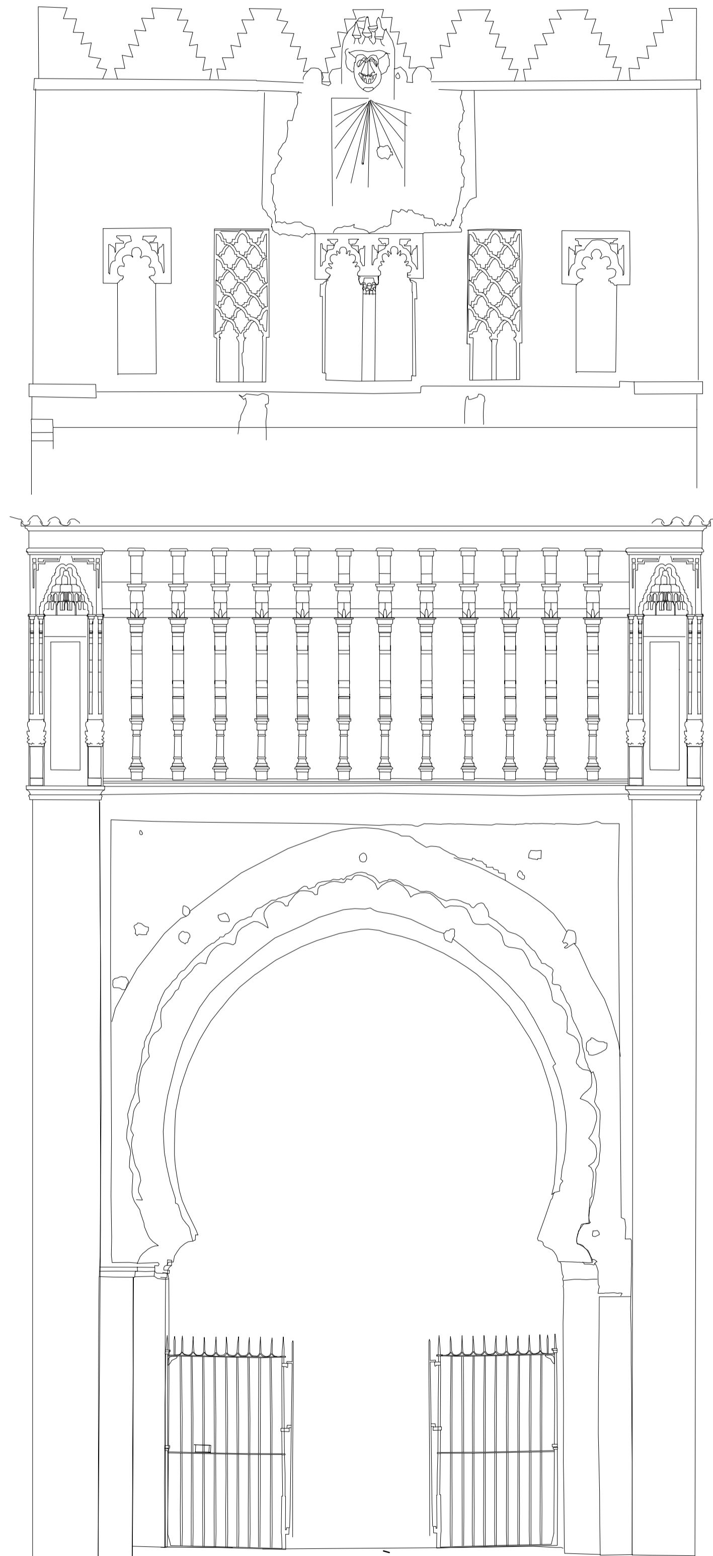
0 1 2 3 m CATEDRAL DE SEVILLA. PUERTA DEL PERDÓN ESQUEMA DE EDIFICIO-GRABES, C.S.C. A. ALMAGRO 1984
