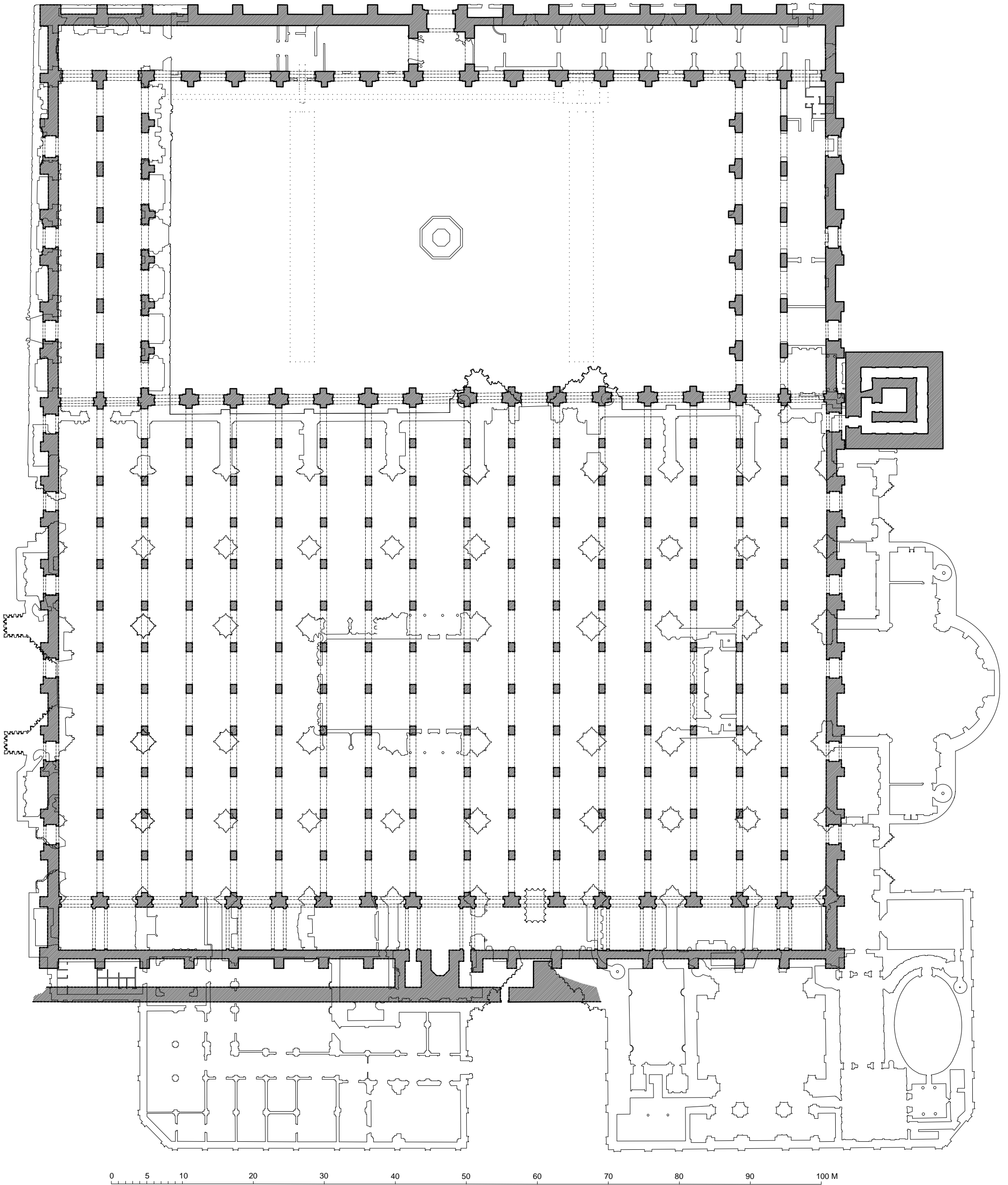
MEZQUITA ALMOHADE DE SEVILLA. PLANTA.
