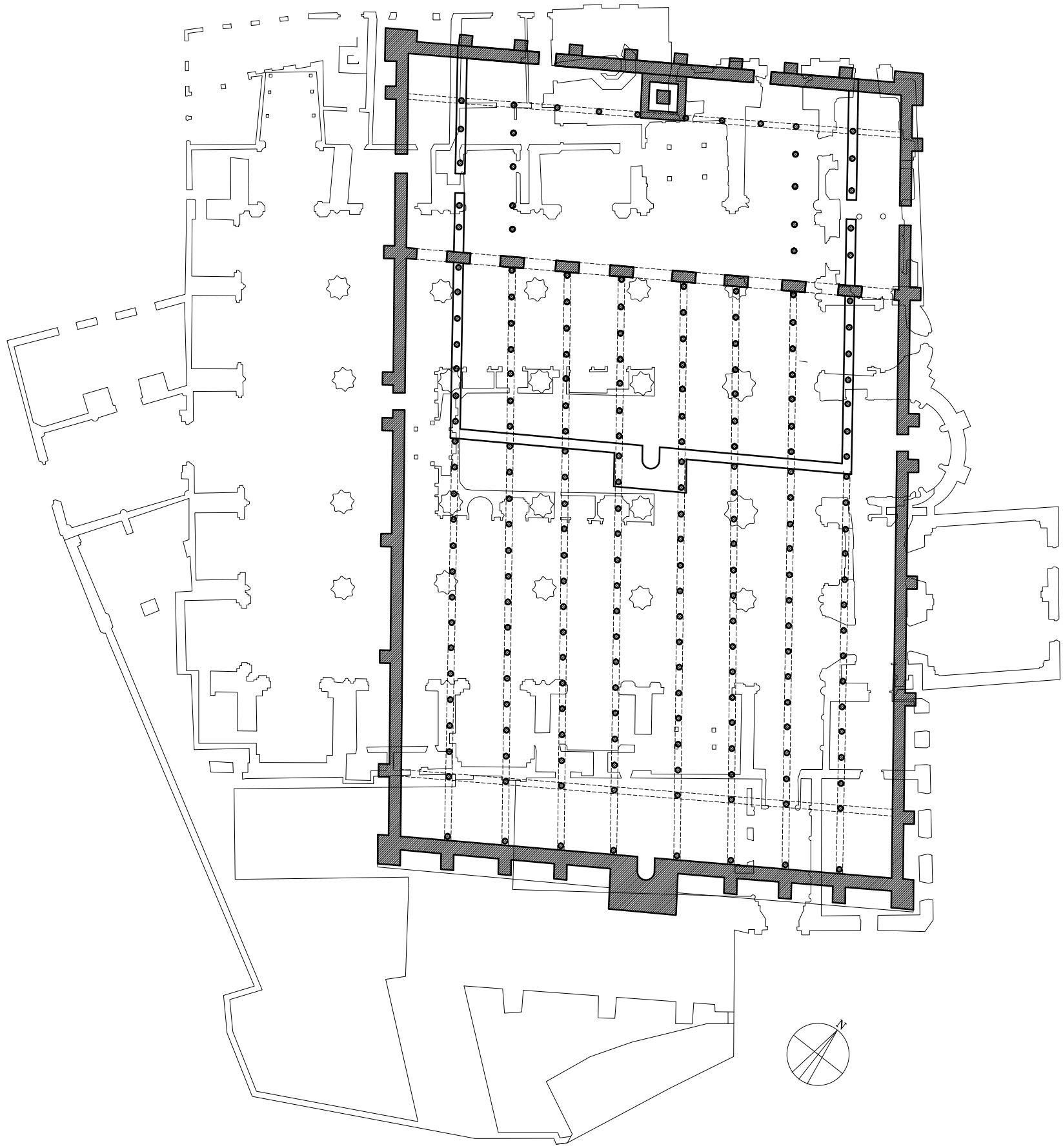
MEZQUITA DE SARAQUSTA. PLANTA. ESCUELA DE ESTUDIOS ARABES. A. ALMAGROCH
