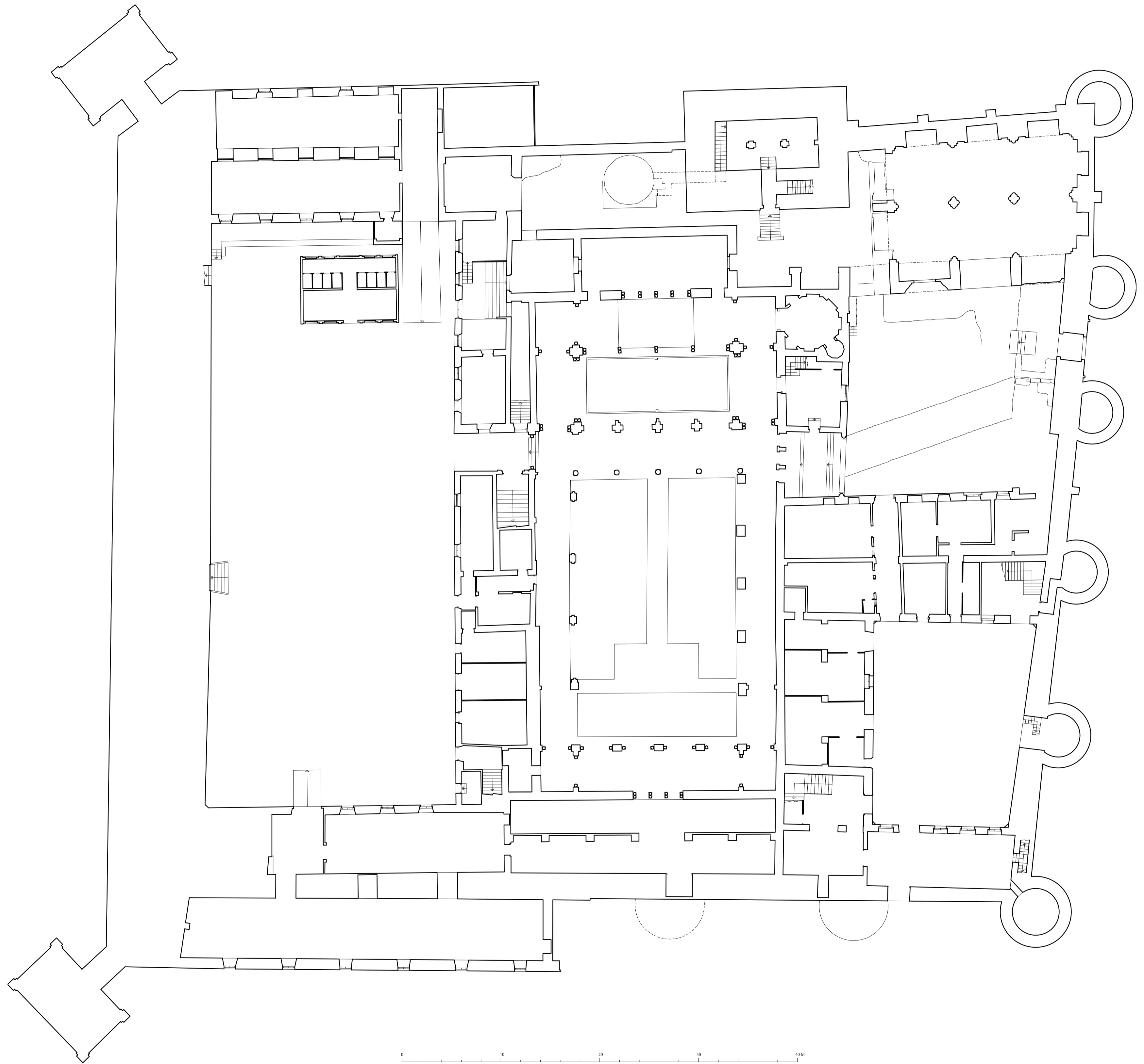
0 10 20 30 40 M LA ALJAFERÍA. ZARAGOZA. PLANTA EN 1980. INSTITUTO DE ESTUDIOS ARABES, C.S.I.C. según el plan de A. Periquetti/1973
