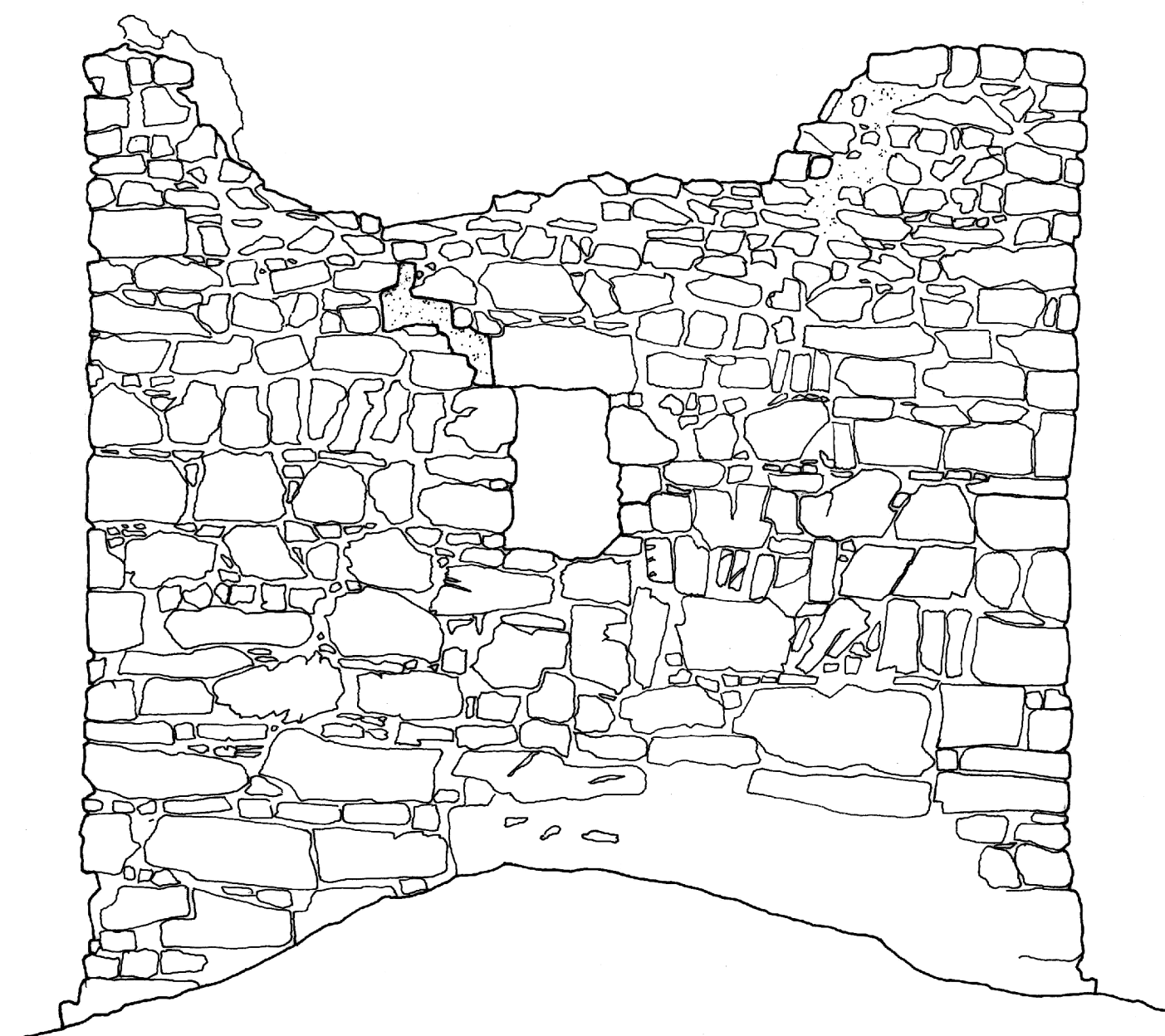
ALZADO NORTE
