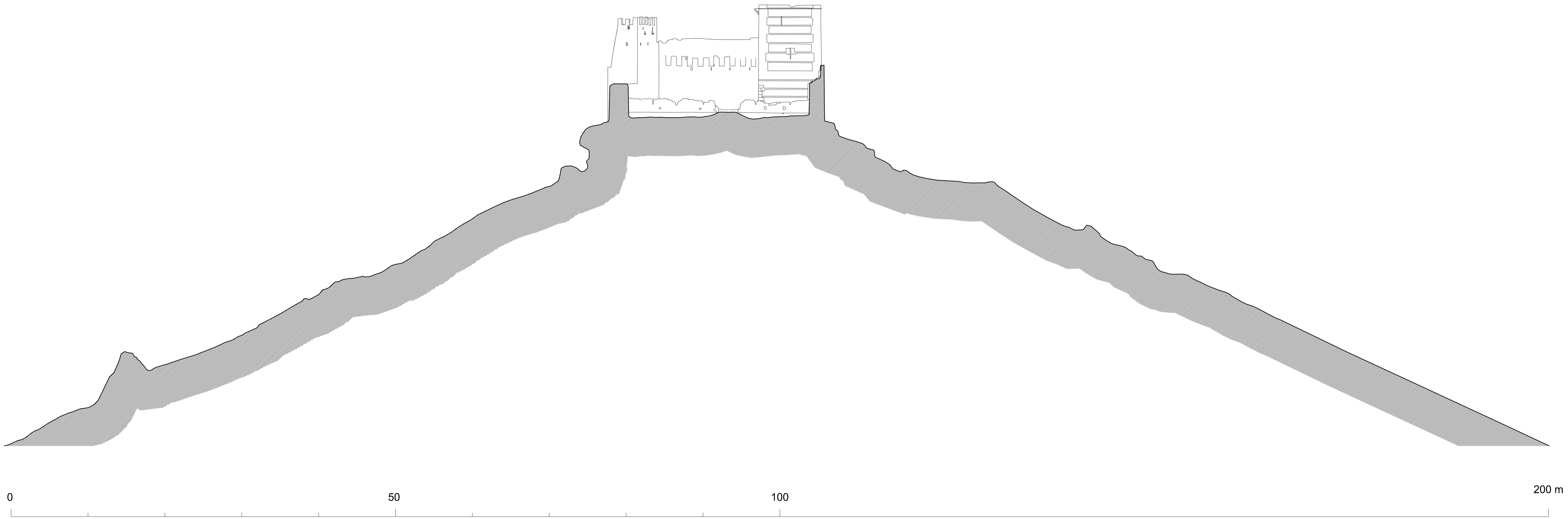
CASTILLO DE GORMAZ (SORIA). SECCION TRANVERSAL
