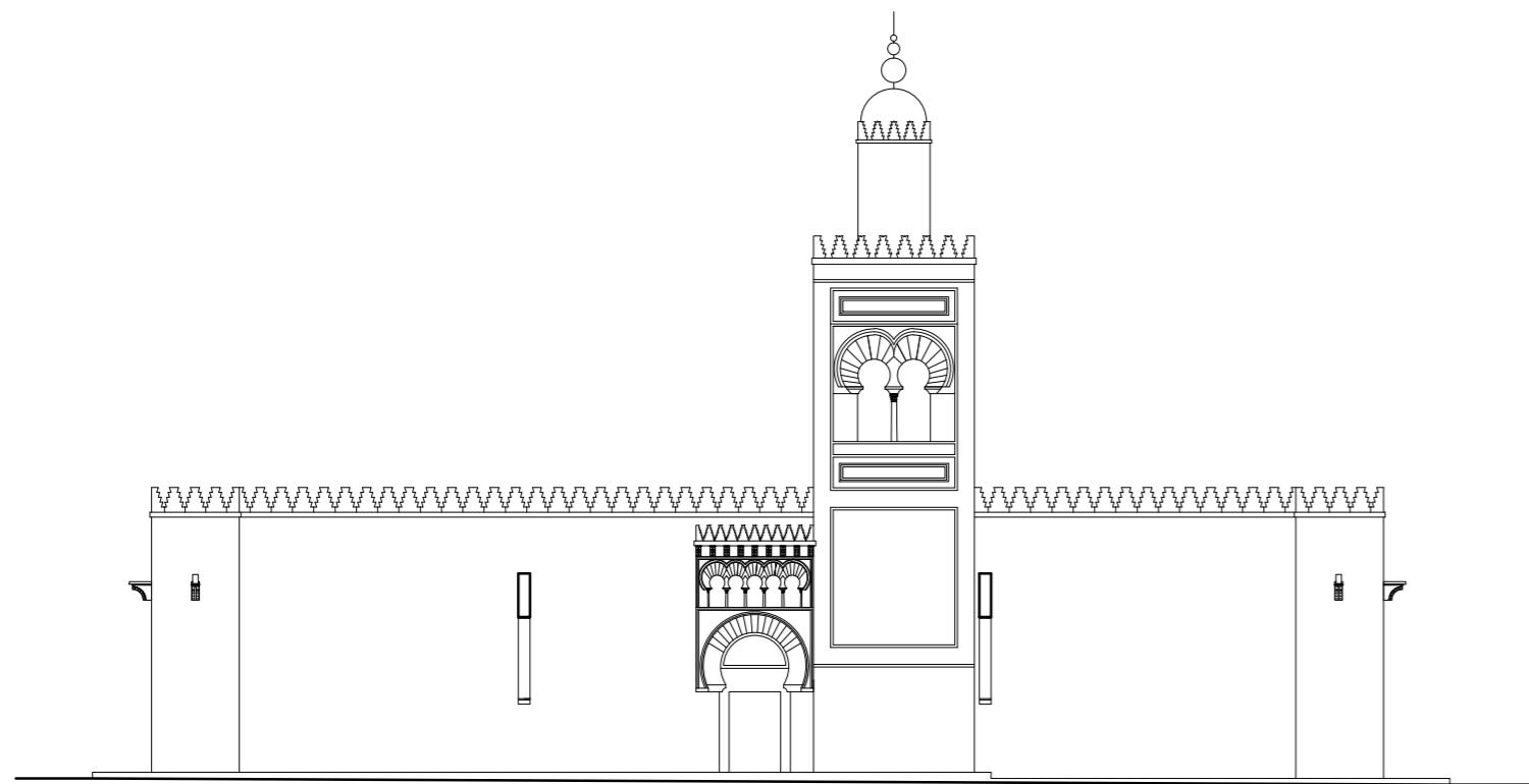
ALZADO A-A
