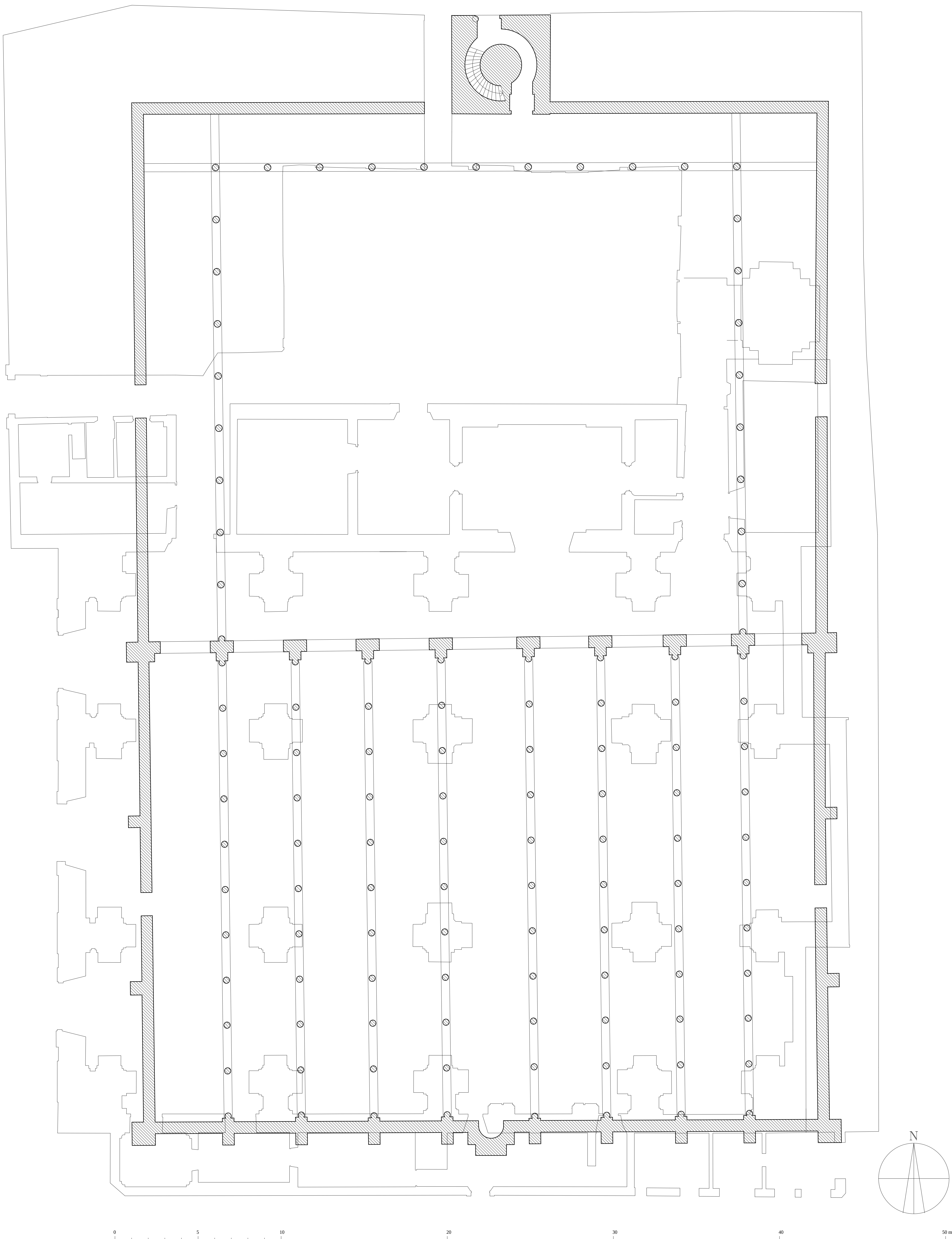
MEZQUITA DE IBN ADABBAS, SEVILLA. PLANTA.
