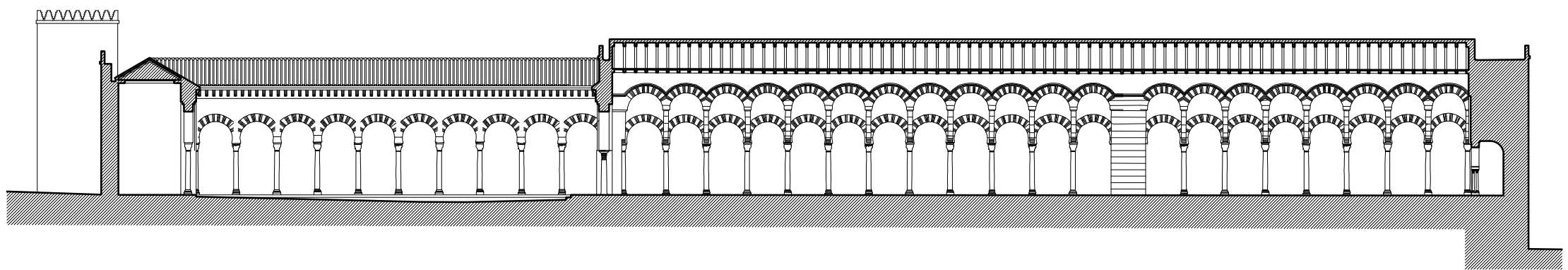
MEZQUITA DE ABD AL-RAHMAN I EN CORDOBA. SECCIÓN LONGITUDINAL HIPÓTESIS A. ALMAGRO 1982.
