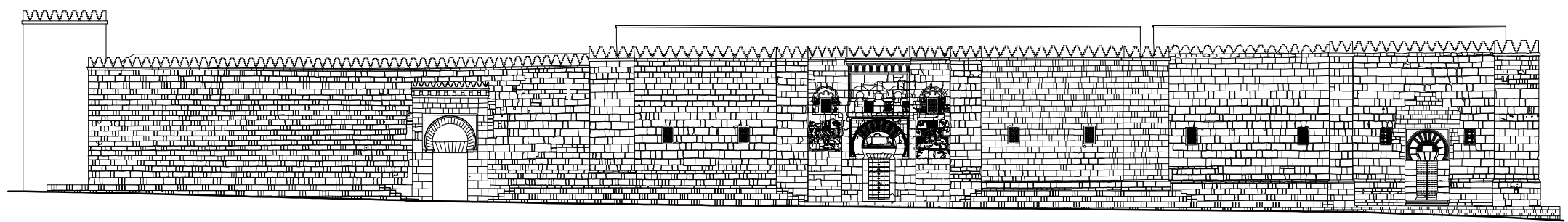
MEZQUITA DE ABD' AL-RAHMAN II EN CORDOBA. ALZADO OESTE. ESCUELA DE ESTUDIOS ARABES, C.S.I.C. A. Almagro / arq. 2014
