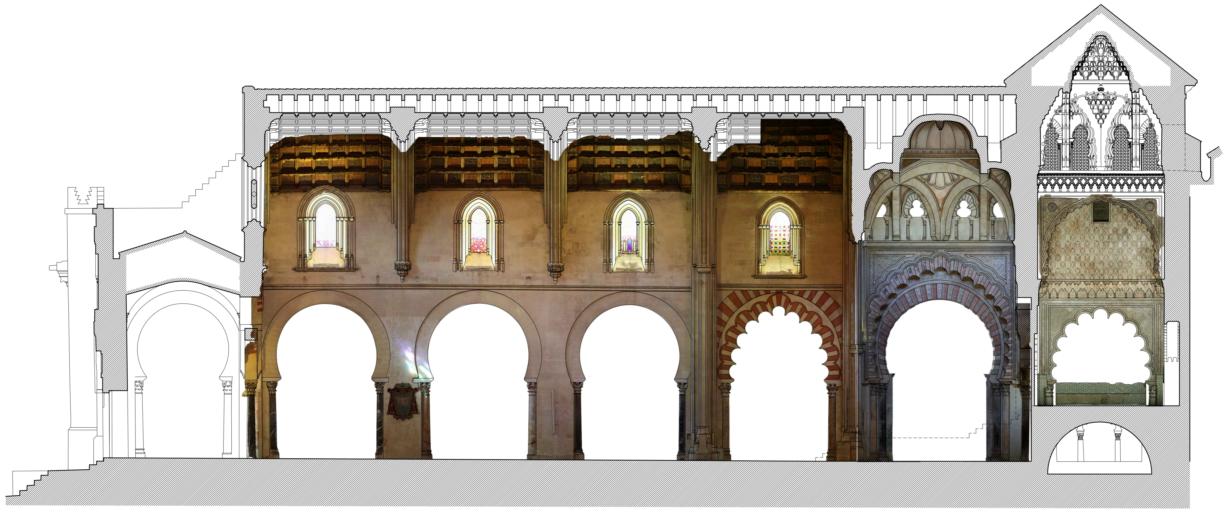
CATEDRAL DE CÓRDOBA. PRIMERA CAPILLA MAYOR, CAPILLA REAL Y NAVE GÓTICA SECCIÓN LONGITUDINAL HACIA NORTE. A. ALMAGRO /ARQ. MARZO 2020
