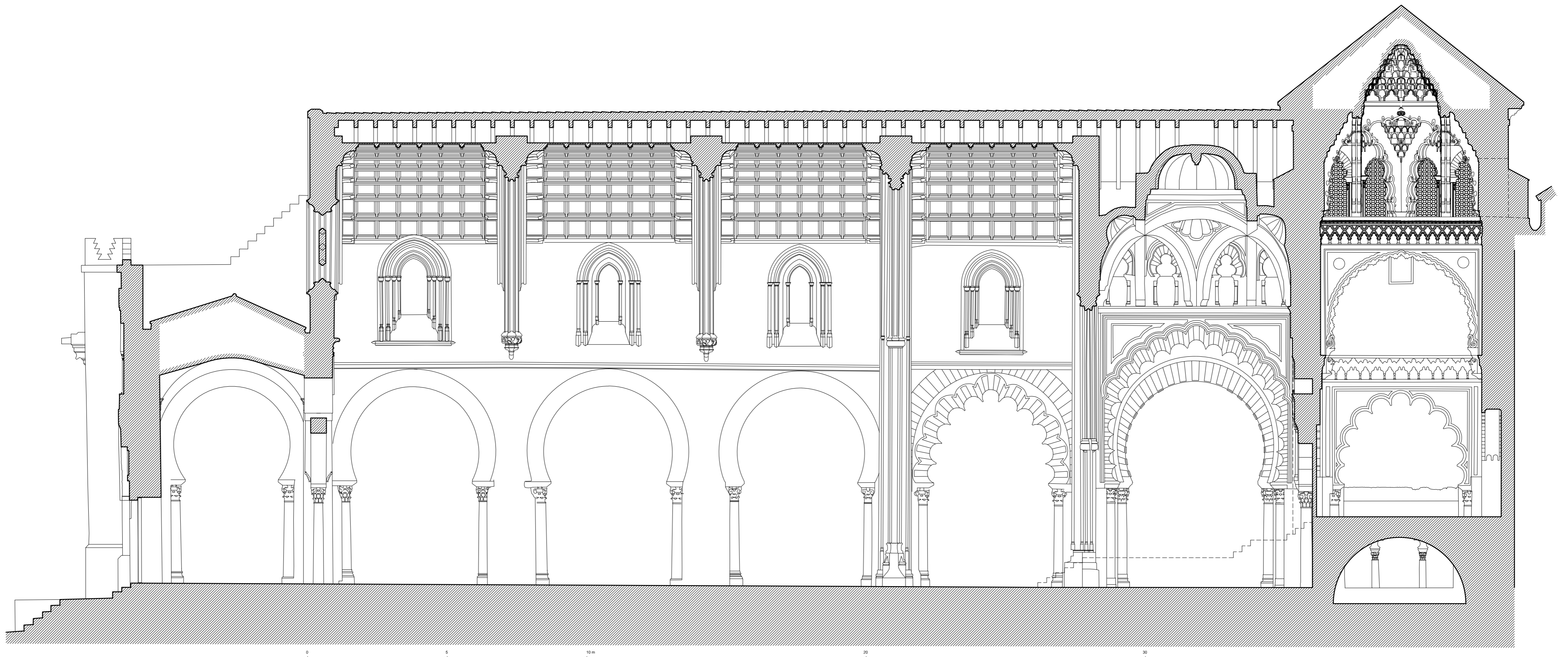
CATEDRAL DE CÓRDOBA. PRIMERA CAPILLA MAYOR, CAPILLA REAL Y NAVE GÓTICA SECCIÓN LONGITUDINAL HACIA NORTE. A. ALMAGRO /ARQ. MARZO 2020
