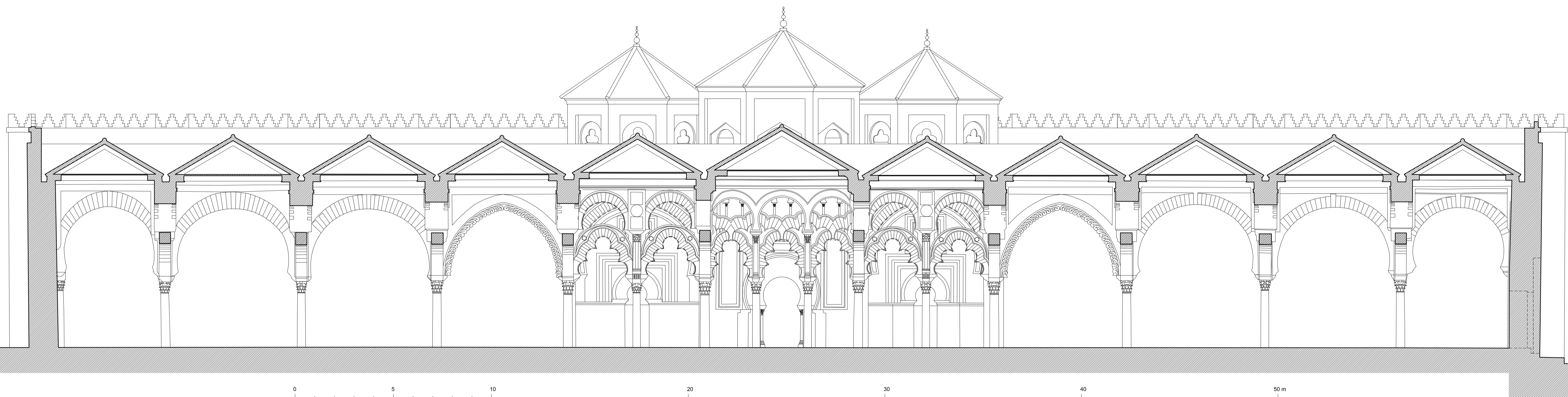
MEZQUITA DE CÓRDOBA. SECCIÓN TRANSVERSAL DE LA AMPLIACIÓN DE AL-HAKAM II CON EL PÓRTICO PARALELO A LA QIBLA DE ALMANZOR A. ALMAGRO IARD. FEBRERO 2020
