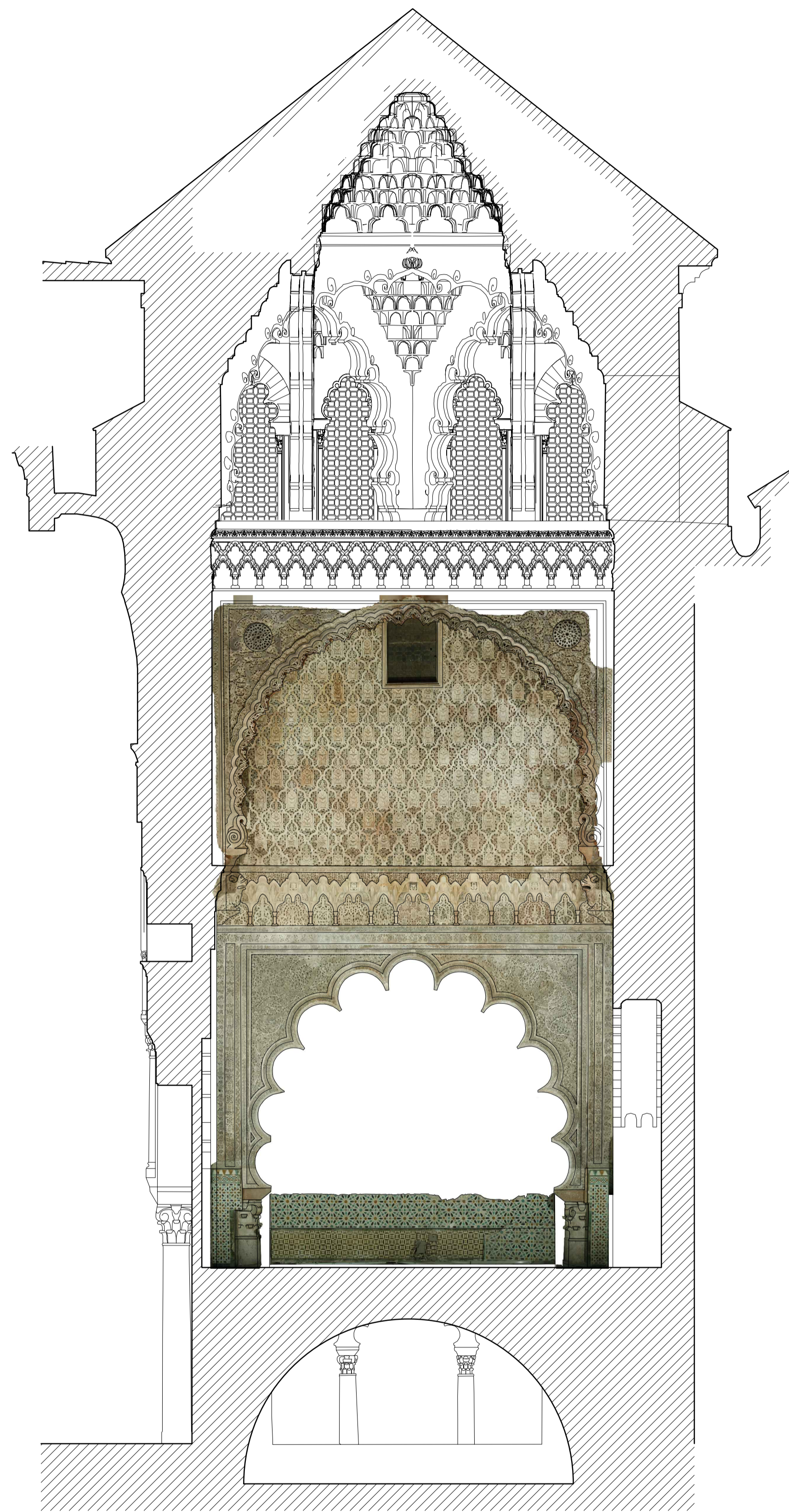
CATEDRAL DE CÓRDOBA. CAPILLA REAL. ALZADOS INTERIORES A. ALMAGRO / ARQ. OCTUBRE 2019
