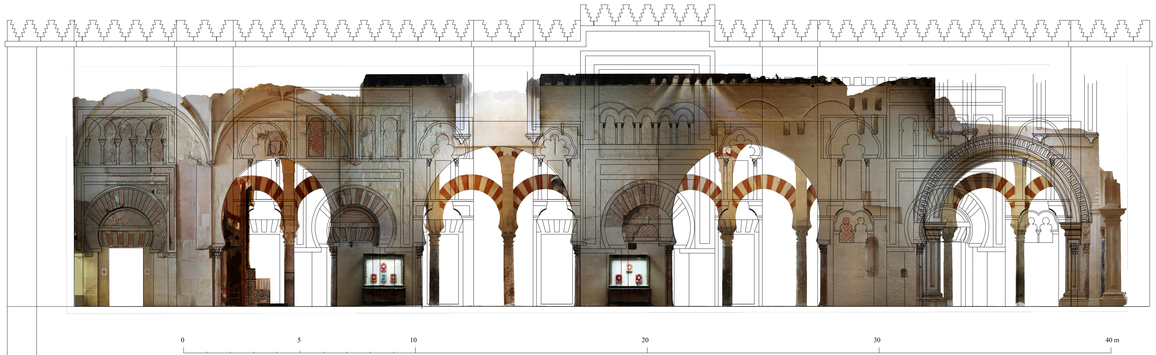
MEZQUITA DE CORDOBA. ALZADO ESTE DE LA AMPLIACION DE AL-HAKAM II A.Almagro / arq. Octubre 2019
