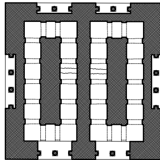
0 5 10 m ALMINAR DE MEZQUITA DE CÓRDOBA. PLANTAS F. HERNÁNDEZ GIMÉNEZ / arq.
