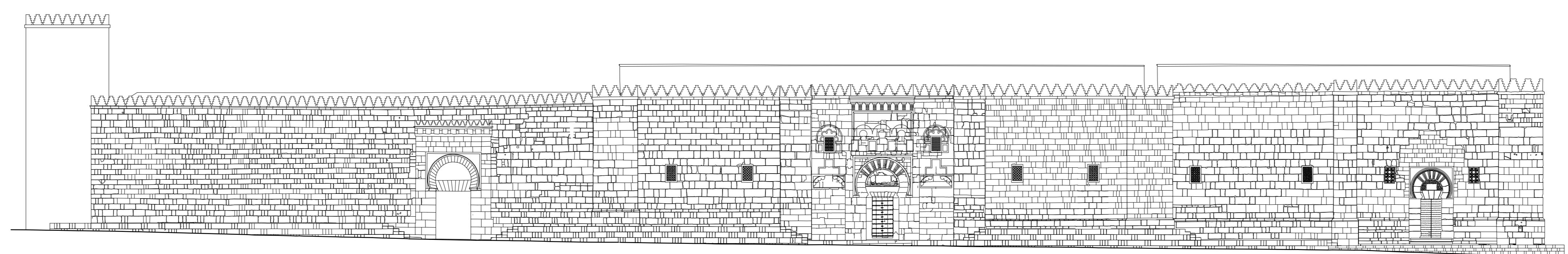
MEZQUITA DE ABD' AL-RAHMAN II EN CORDOBA. ALZADO OESTE.
