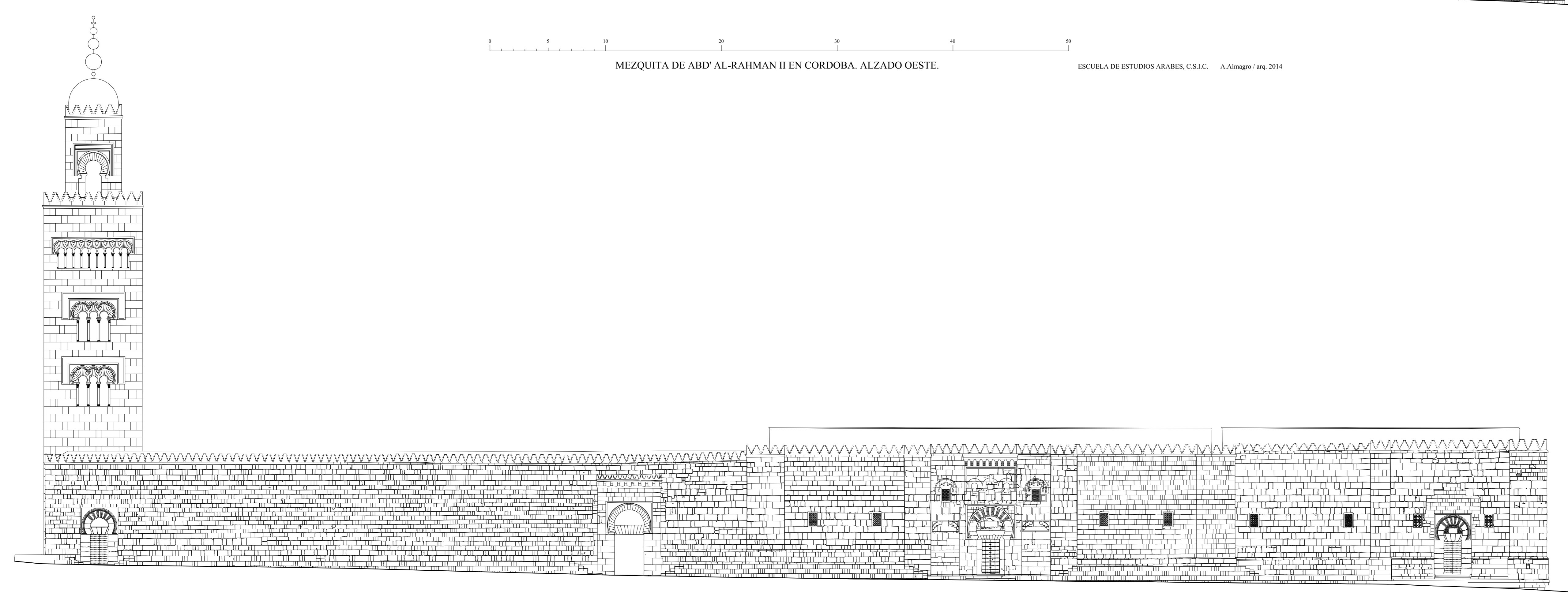
MEZQUITA DE ABD' AL-RAHMAN III EN CORDOBA. ALZADO OESTE.
