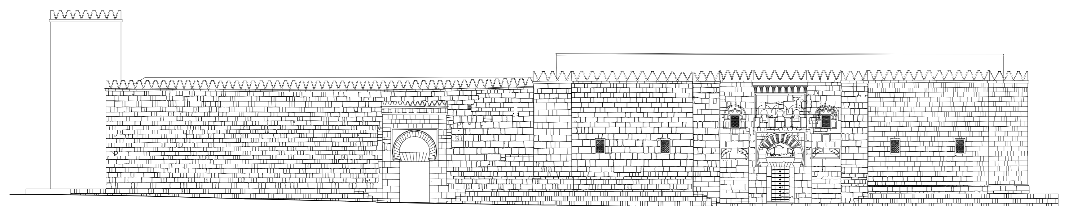
MEZQUITA DE ABD' AL-RAHMAN I EN CORDOBA. ALZADO OESTE.
