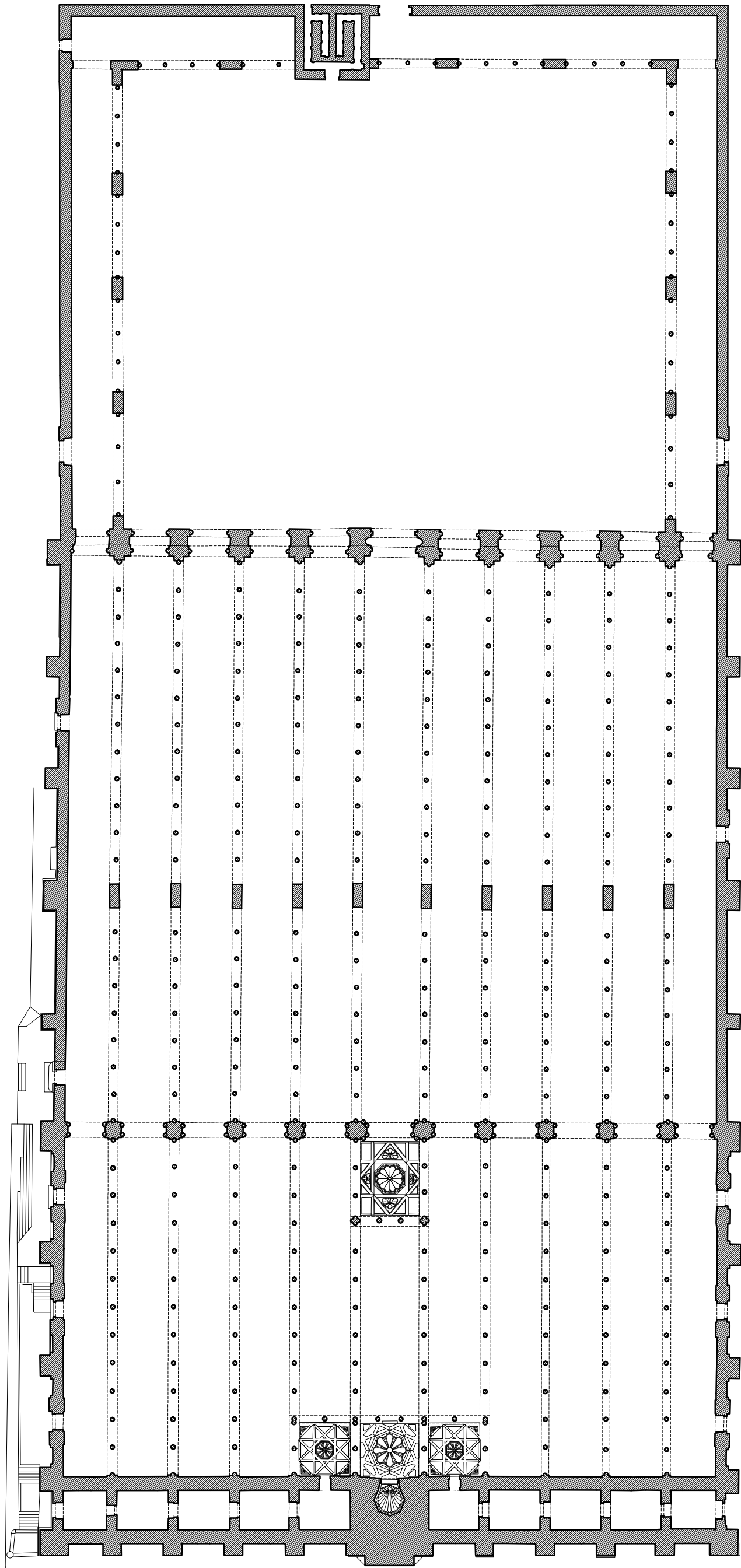
MEZQUITA DE CÓRDOBA. Siglo X ESCUELA DE ESTUDIOS ÁRABES, CSIC. A. ALMAGRO / arq.
